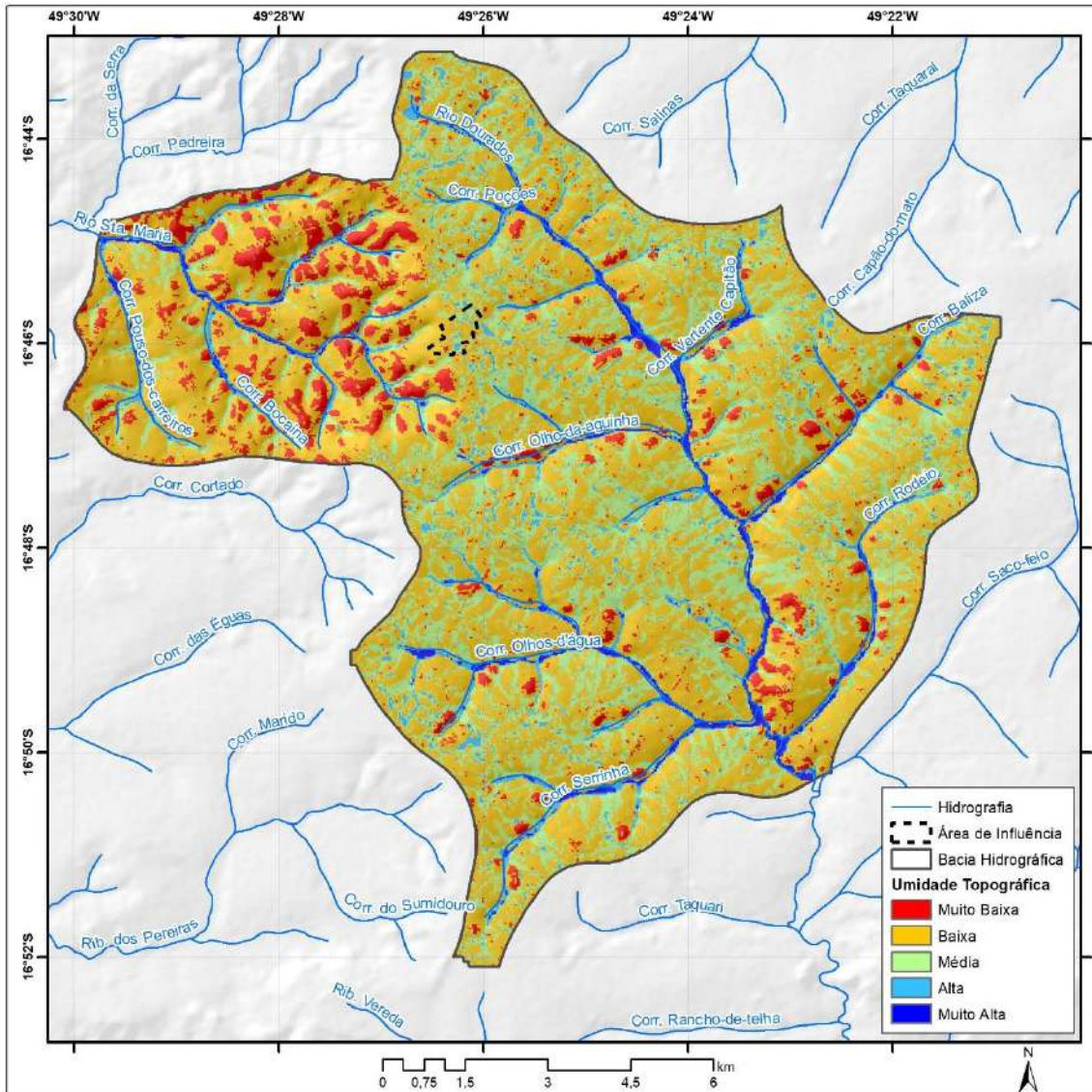
Mapa 3.10 – Índice de umidade topográfica na bacia hidrográfica do rio Dourados e na área de influência da Comunidade Recantos Dourados, Abadia de Goiás-GO, 2020.
