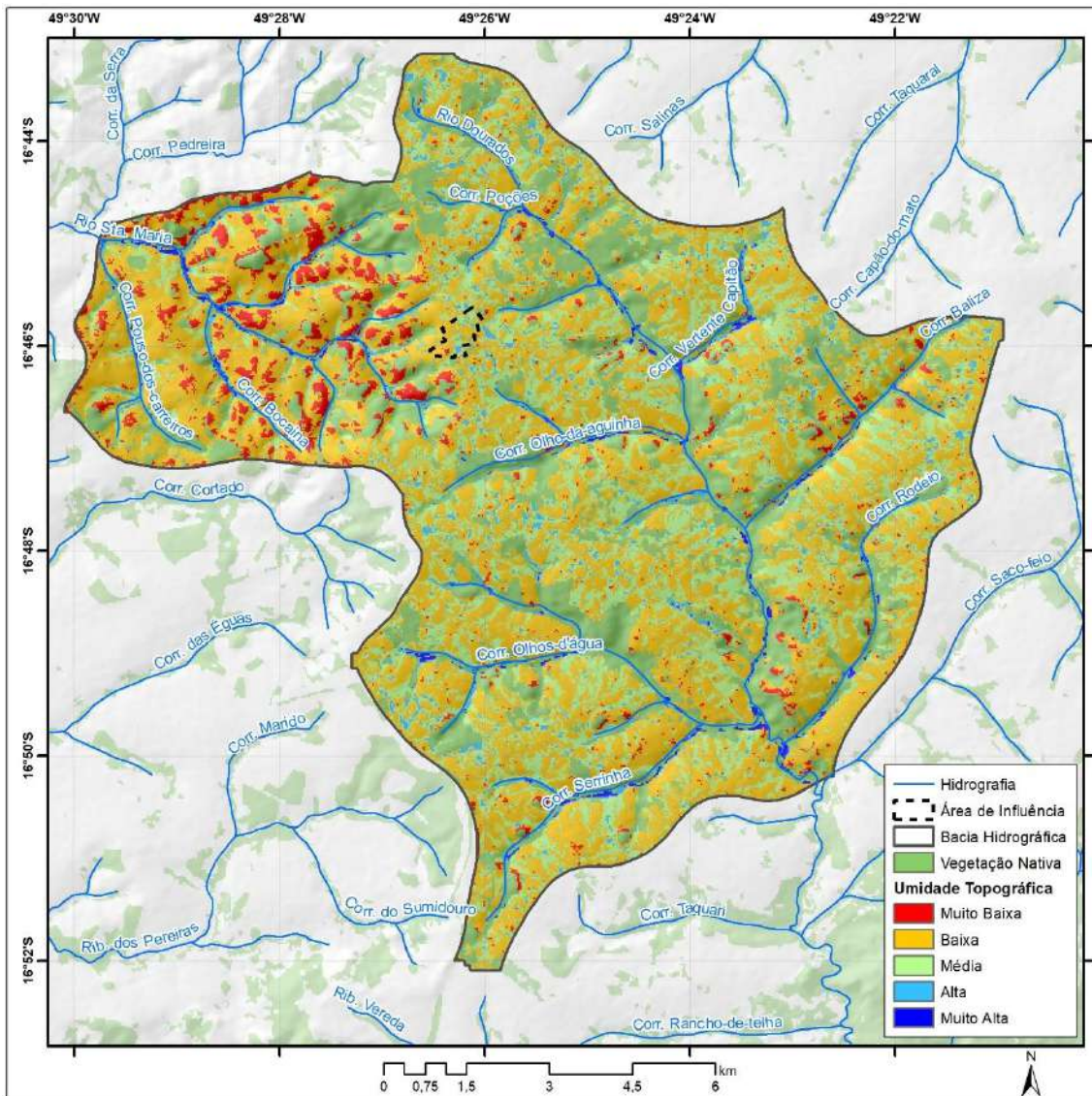
Mapa 3.11 – Índice de umidade topográfica e cobertura de vegetação nativa remanescente na bacia hidrográfica do rio Dourados e da área de influência da Comunidade Recantos Dourados, Abadia de Goiás-GO, 2020.
