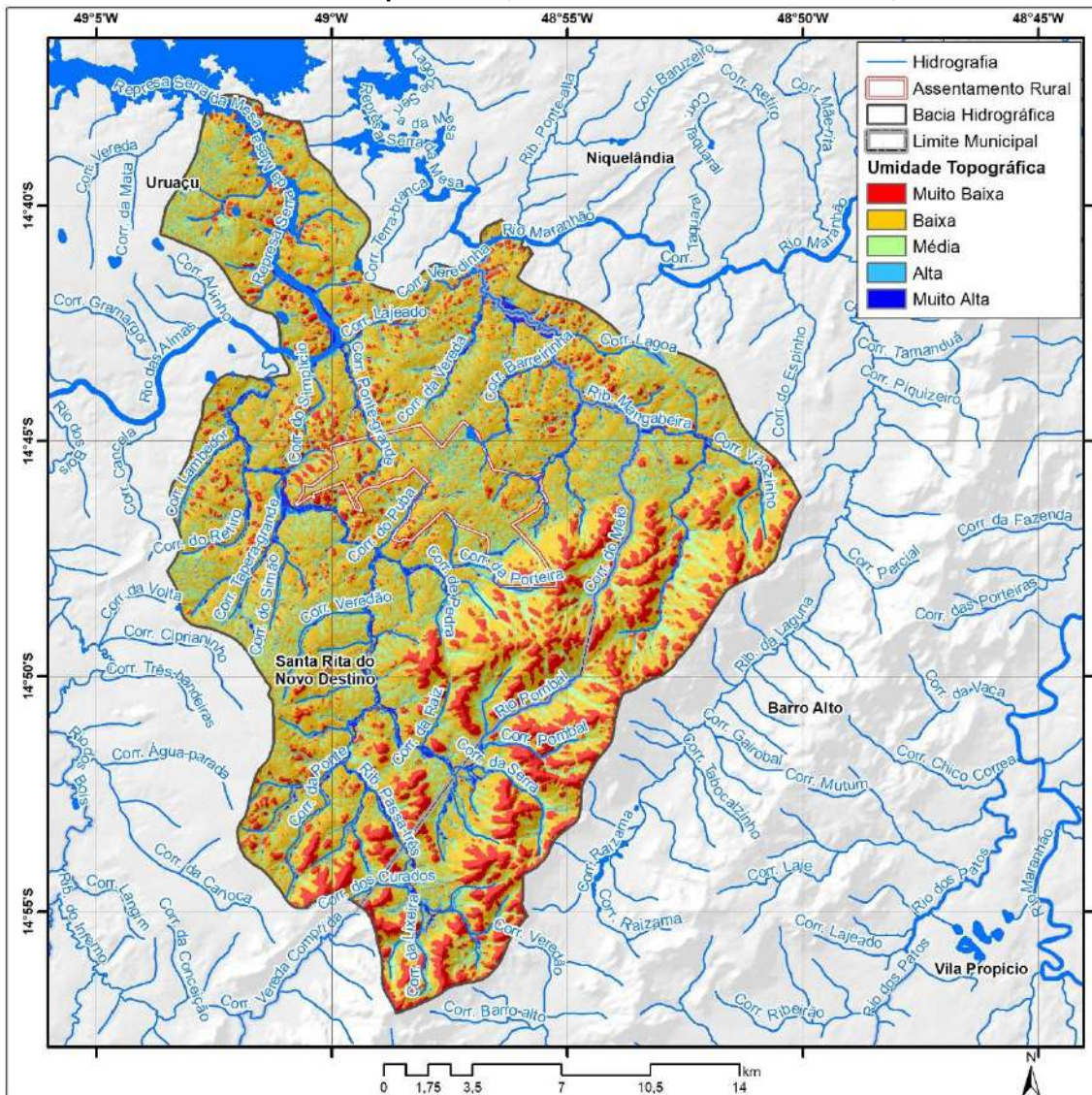
Mapa 3.10 – Índice de umidade topográfica na foz da bacia hidrográfica do rio das Almas e do assentamento da Comunidade Independência, Santa Rita do Novo Destino-GO, 2020.
