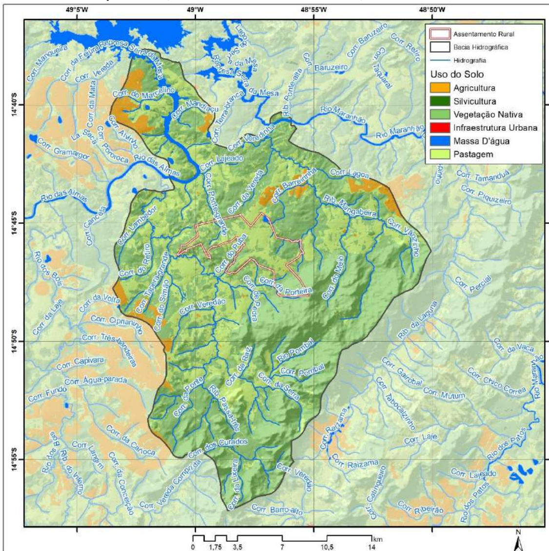
Mapa 3.3 – Cobertura e uso do solo na foz da bacia hidrográfica do rio das Almas e do assentamento da Comunidade Independência, Santa Rita do Novo Destino-GO, 2020.
