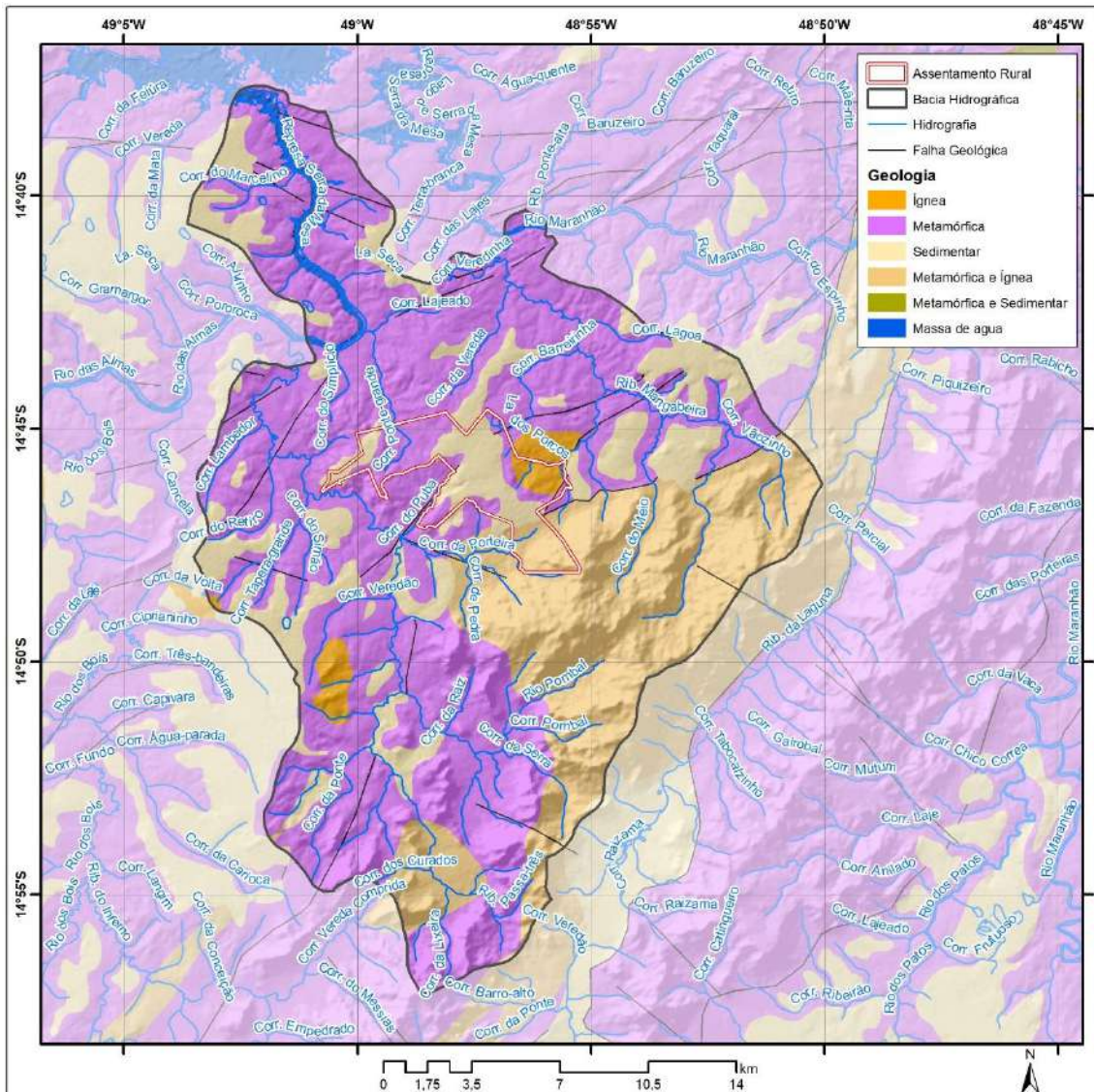
Mapa 3.4 – Litologia da foz da bacia hidrográfica do rio das Almas e do assentamento da Comunidade Independência, Santa Rita do Novo Destino-GO, 2020.
