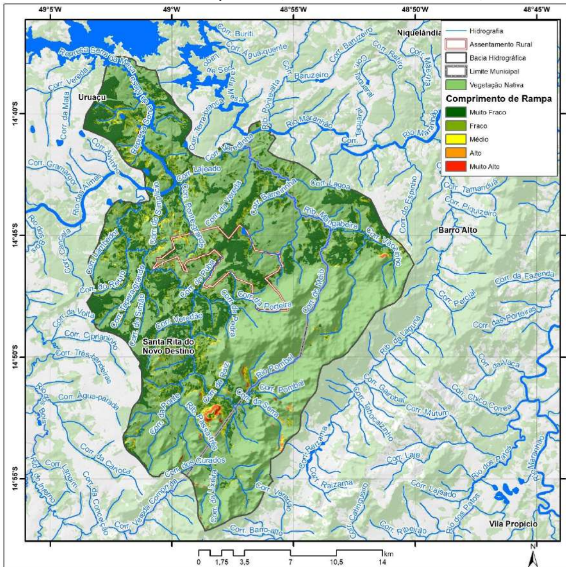
Mapa 3.9 – Cobertura de vegetação nativa no relevo da foz da bacia hidrográfica do rio das Almas e do assentamento da Comunidade Independência, Santa Rita do Novo Destino-GO, 2020.
