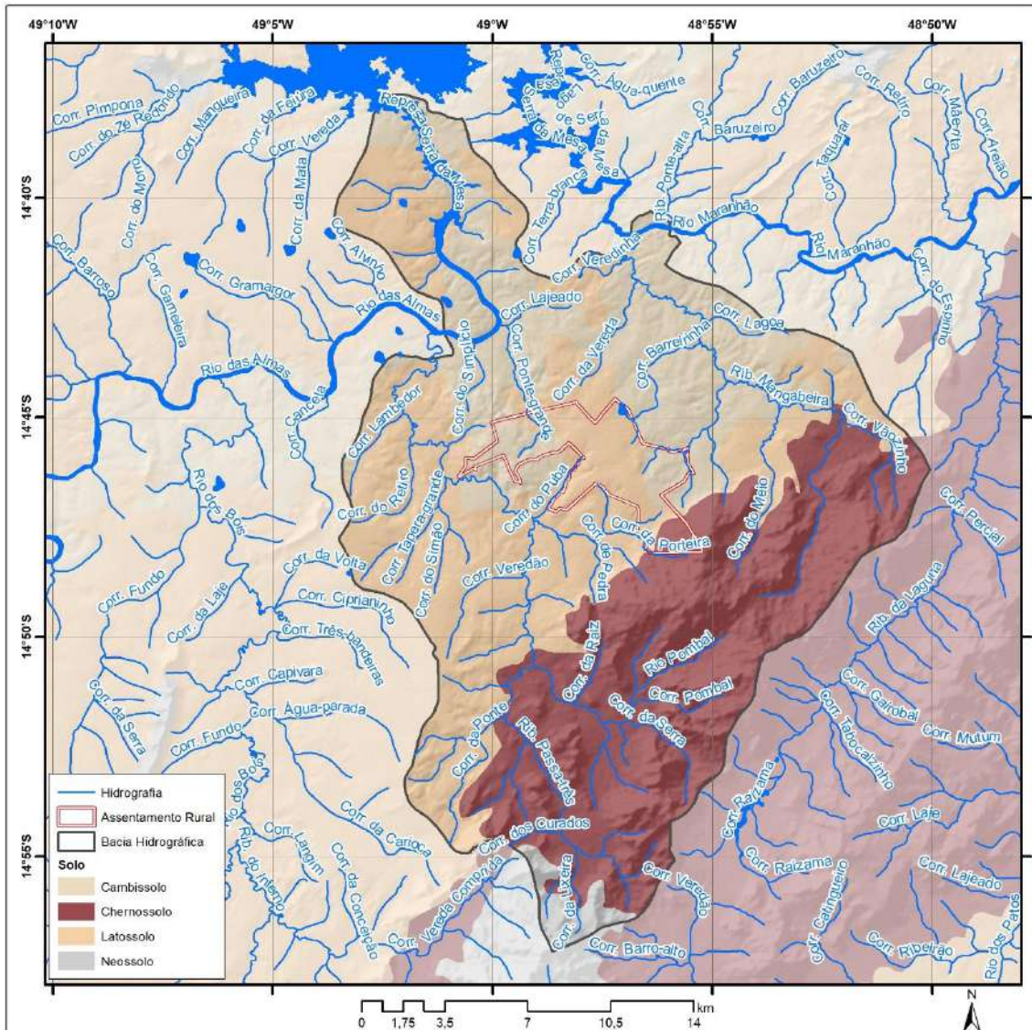
Mapa 3.7 – Tipo de solo da foz da bacia hidrográfica do rio das Almas e do assentamento da Comunidade Independência, Santa Rita do Novo Destino-GO, 2020.
