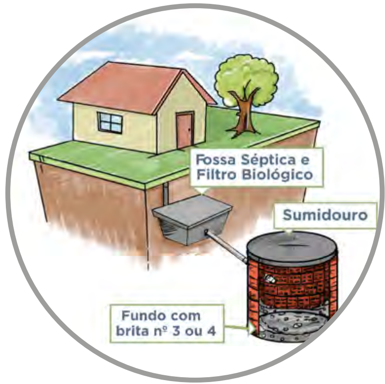
Fossa séptica
