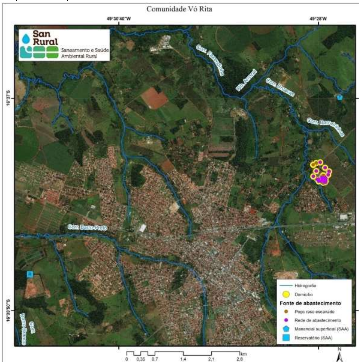
Mapa 6.1 – Distribuição espacial dos domicílios e sua fonte de abastecimento de água, juntamente com o respectivo ponto de captação e o reservatório de distribuição do SAA, na Comunidade de Vó Rita, Trindade-GO, 2019.
