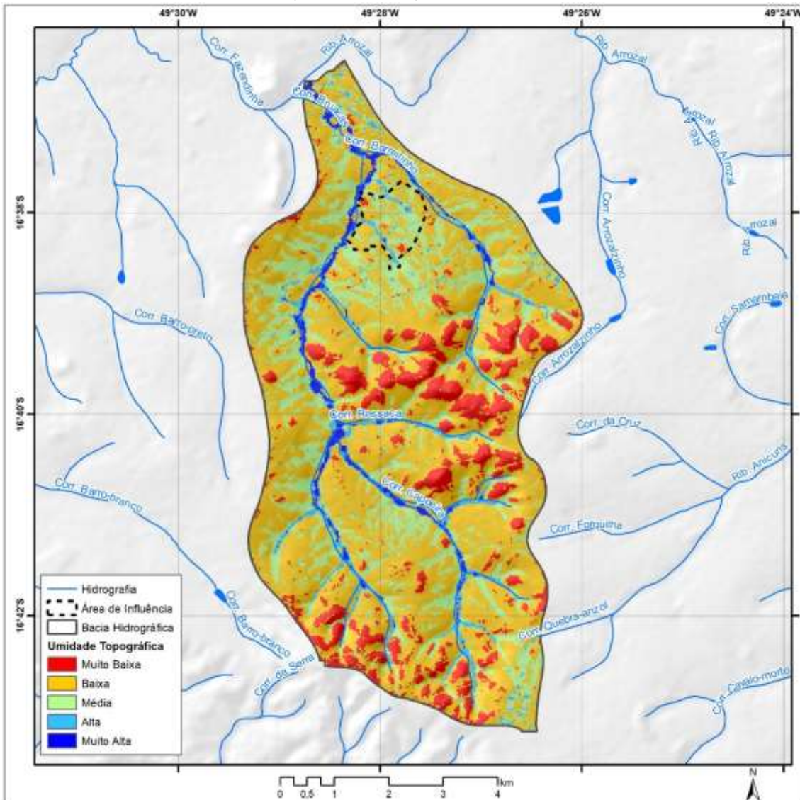
Mapa 3.10 – Índice de umidade topográfica na bacia hidrográfica do córrego Bruacas e da área de influência da Comunidade de Vó Rita, Trindade-GO, 2020.
