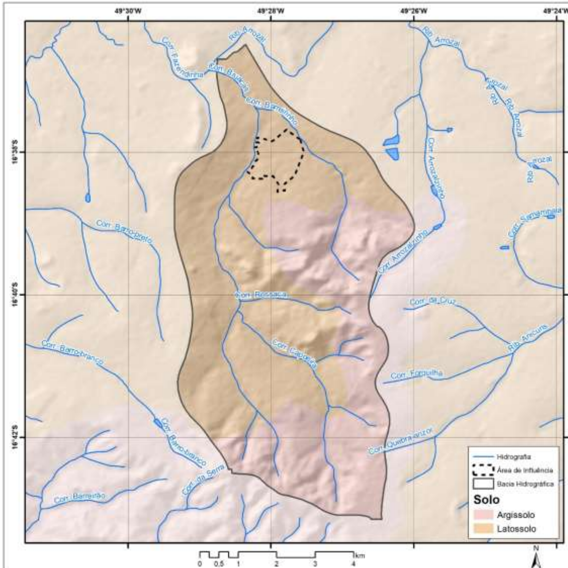
Mapa 3.7 – Tipo de solo da bacia hidrográfica do córrego Bruacas e da área de influência da Comunidade de Vó Rita, Trindade-GO, 2020.
