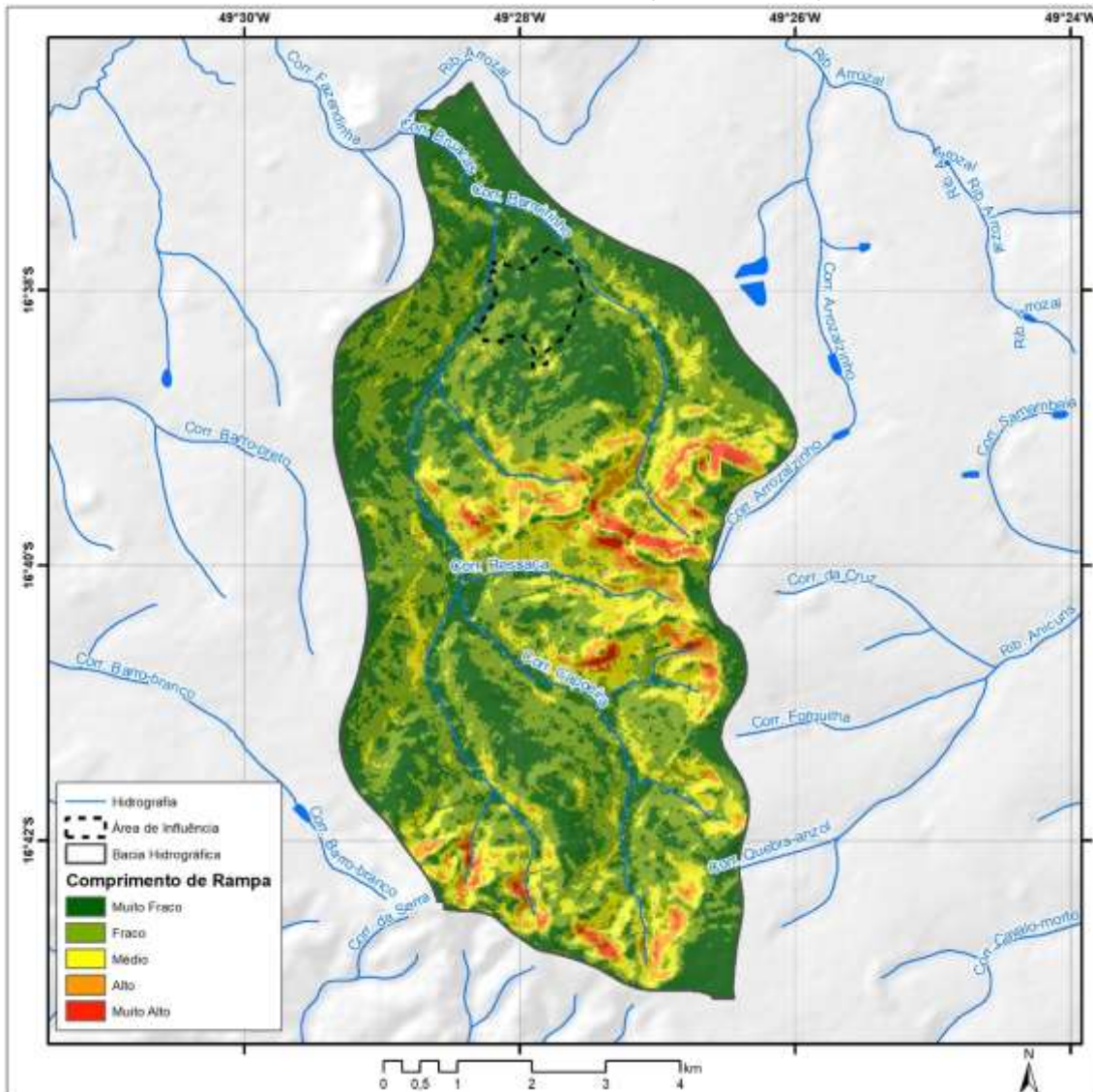
Mapa 3.8 – Comprimento de rampas de declividade do relevo na bacia hidrográfica do córrego Bruacas e da área de influência da Comunidade de Vó Rita, Trindade-GO, 2020.
