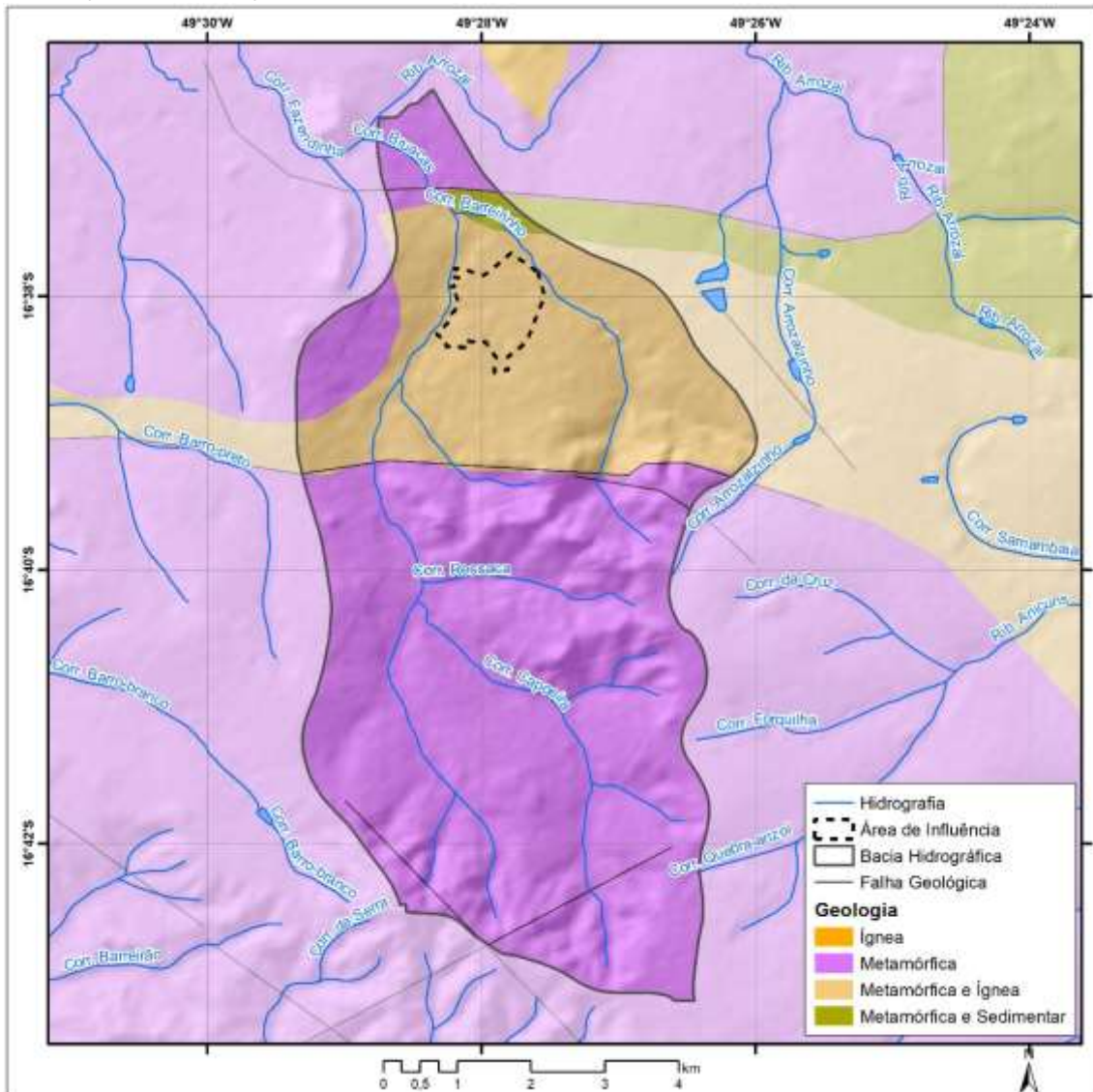
Mapa 3.4 – Litologia da bacia hidrográfica do córrego Bruacas e da área de influência da Comunidade de Vó Rita, Trindade-GO, 2020.
