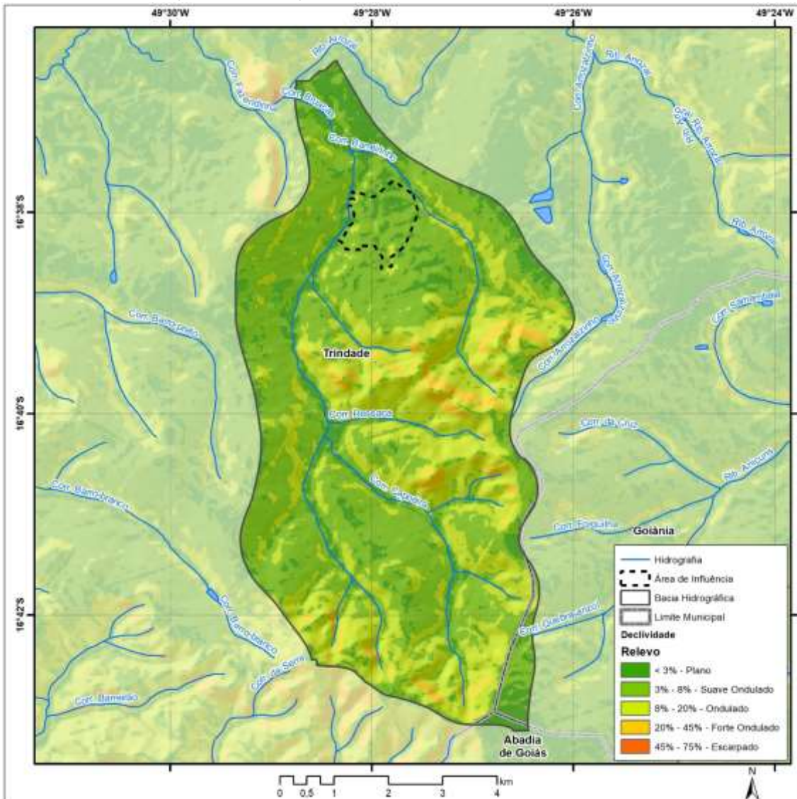
Mapa 3.6 – Declividade da bacia hidrográfica do córrego Bruacas e da área de influência da Comunidade de Vó Rita, Trindade-GO, 2020.
