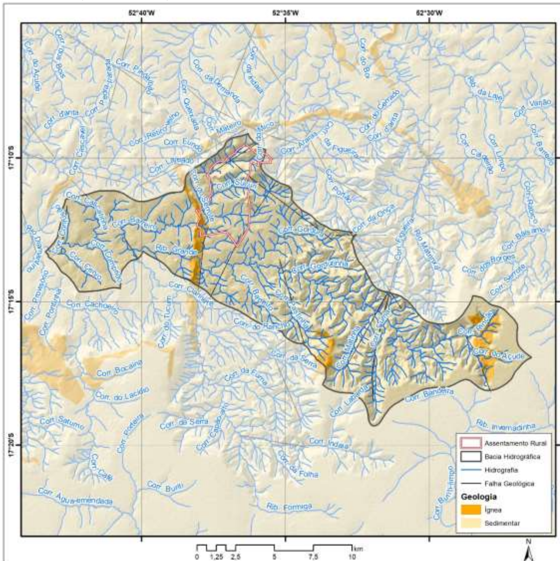
Mapa 3.4 – Litologia da bacia hidrográfica do ribeirão Grande e do assentamento da Comunidade Serra das Araras, Mineiros-GO, 2020.
