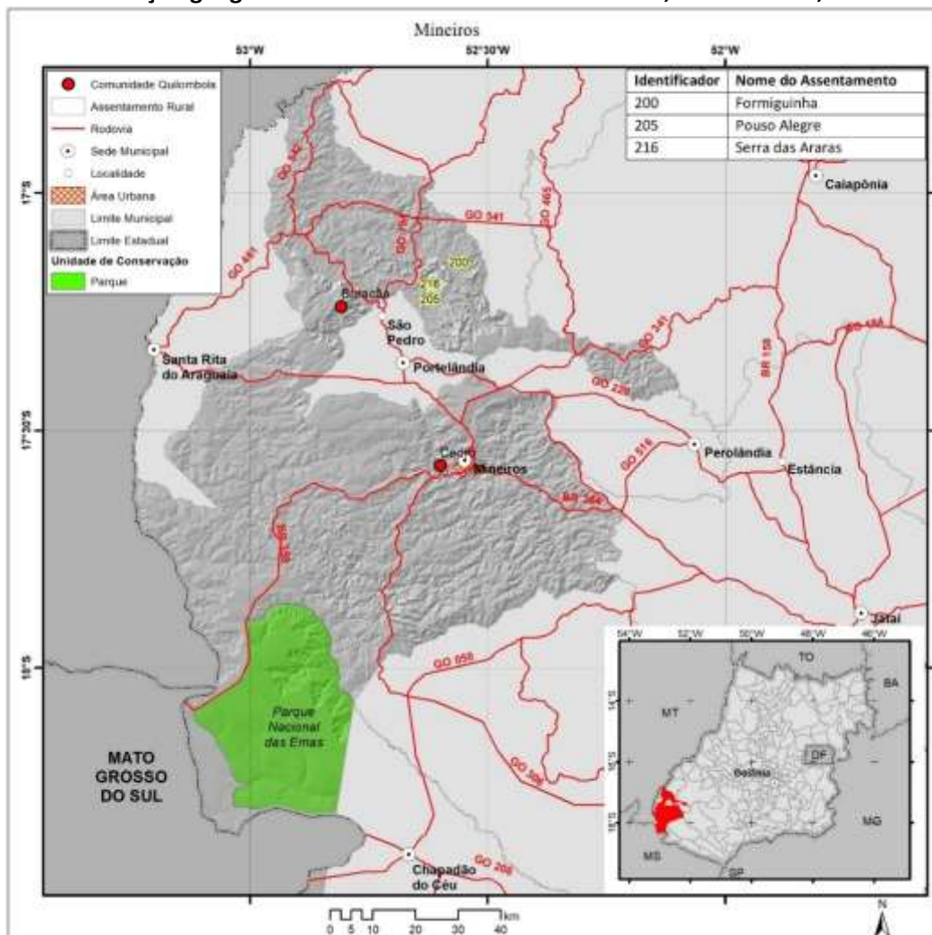
Mapa 3.1 – Localização geográfica da Comunidade Serra das Araras, Mineiros-GO, 2020.
