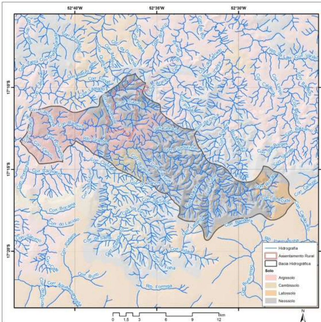
Mapa 3.7 – Tipo de solo da bacia hidrográfica do ribeirão Grande e do assentamento da Comunidade Serra das Araras, Mineiros-GO, 2020.
