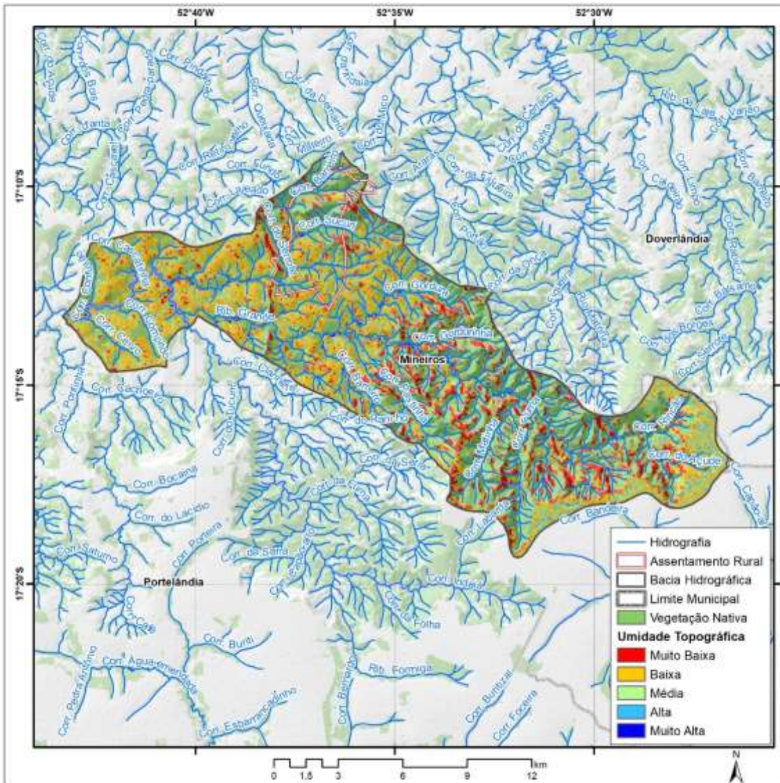
Mapa 3.11 – Índice de umidade topográfica e cobertura de vegetação nativa remanescente na bacia hidrográfica do ribeirão Grande e do assentamento da Comunidade Serra das Araras, Mineiros-GO, 2020.
