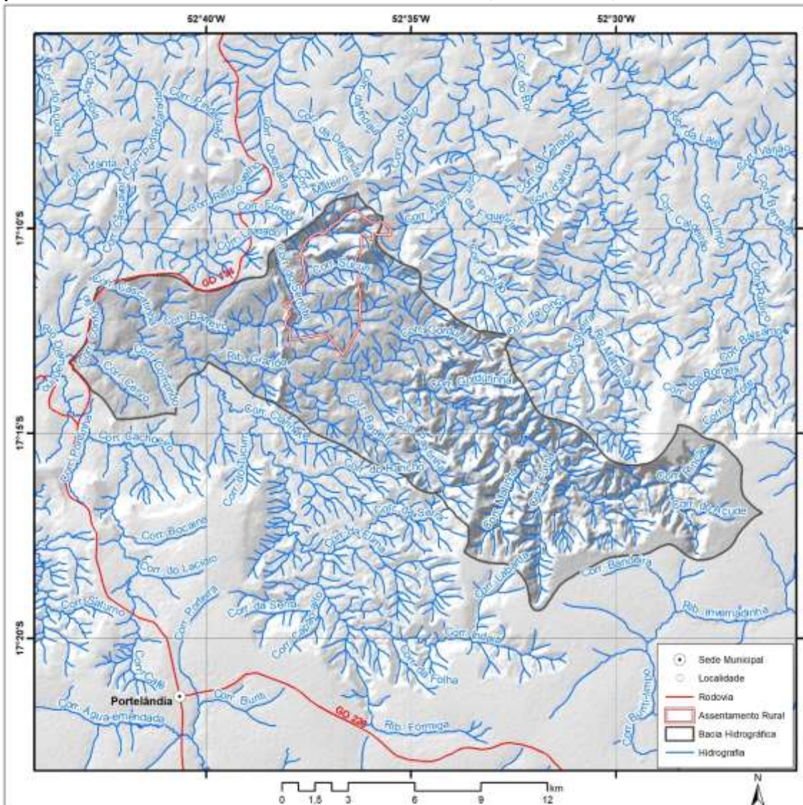
Mapa 3.2 – Assentamento da Comunidade Serra das Araras, Mineiros-GO, 2020.
