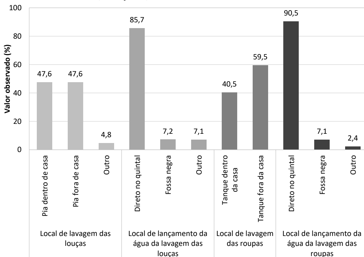
Gráfico 6.5 – Localização dos aparelhos hidrossanitários e locais de geração e de lançamento da água cinza, proveniente da pia para lavagem das louças, e do tanque para lavagem das roupas, na Comunidade São Salvador, Minaçu-GO, 2018.
