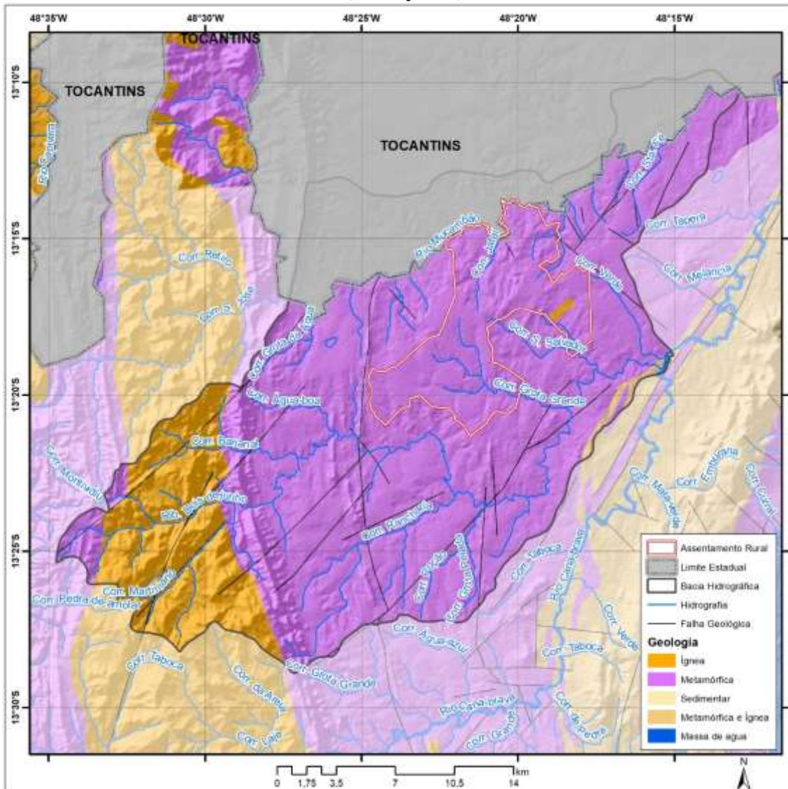
Mapa 3.4 – Litologia das bacias hidrográficas do rio Mucambão e do córrego São Salvador e do assentamento da Comunidade São Salvador, Minaçu-GO, 2020.
