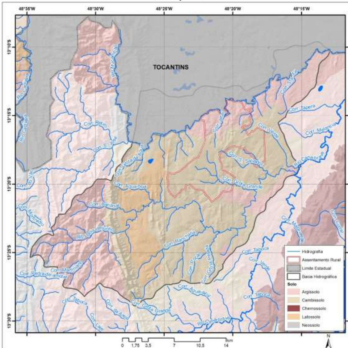
Mapa 3.7 – Tipo de solo das bacias hidrográficas do rio Mucambão e do córrego São Salvador e do assentamento da Comunidade São Salvador, Minaçu-GO, 2020.
