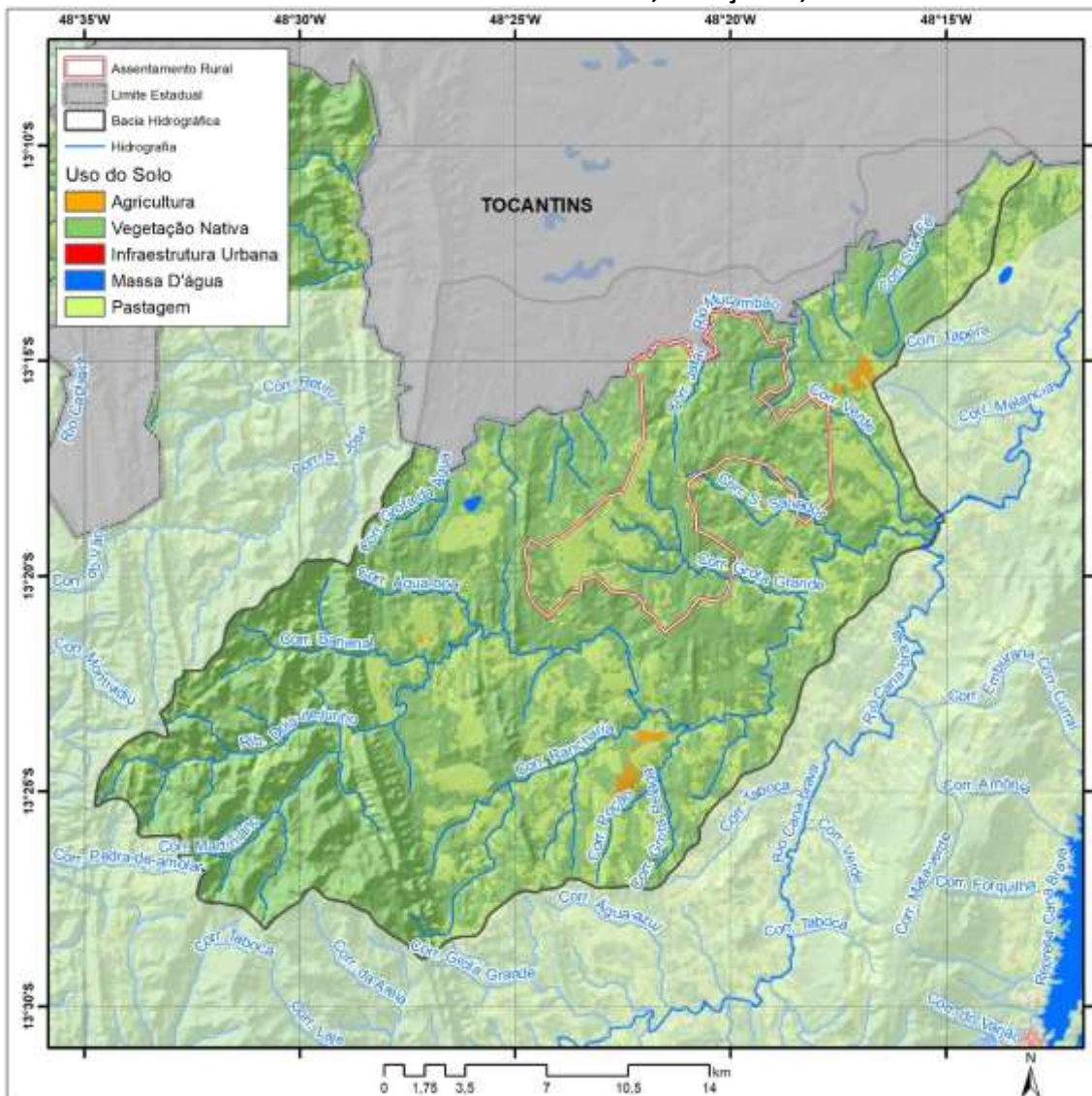
Mapa 3.3 – Cobertura e uso do solo nas bacias hidrográficas do rio Mucambão e do córrego São Salvador e do assentamento da Comunidade São Salvador, Minaçu-GO, 2020.
