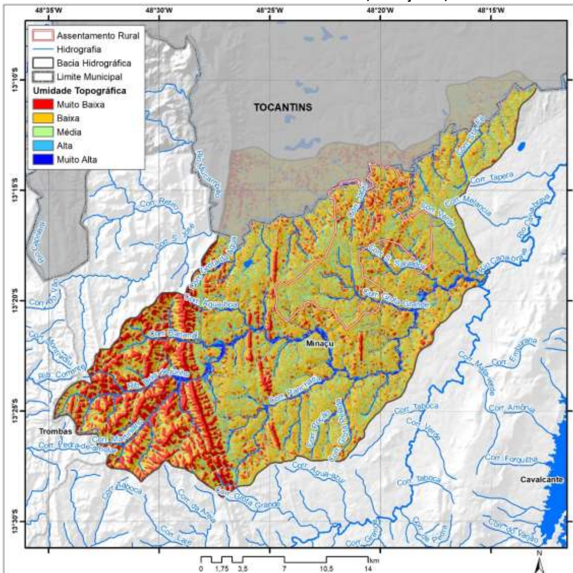
Mapa 3.10 – Índice de umidade topográfica nas bacias hidrográficas do rio Mucambão e do córrego São Salvador e do assentamento da Comunidade São Salvador, Minaçu-GO, 2020.
