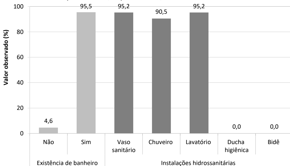
Gráfico 6.5 – Tipos de aparelhos hidrossanitários existentes nos banheiros das unidades familiares da Comunidade Salto para o Futuro, Niquelândia-GO, 2018.
