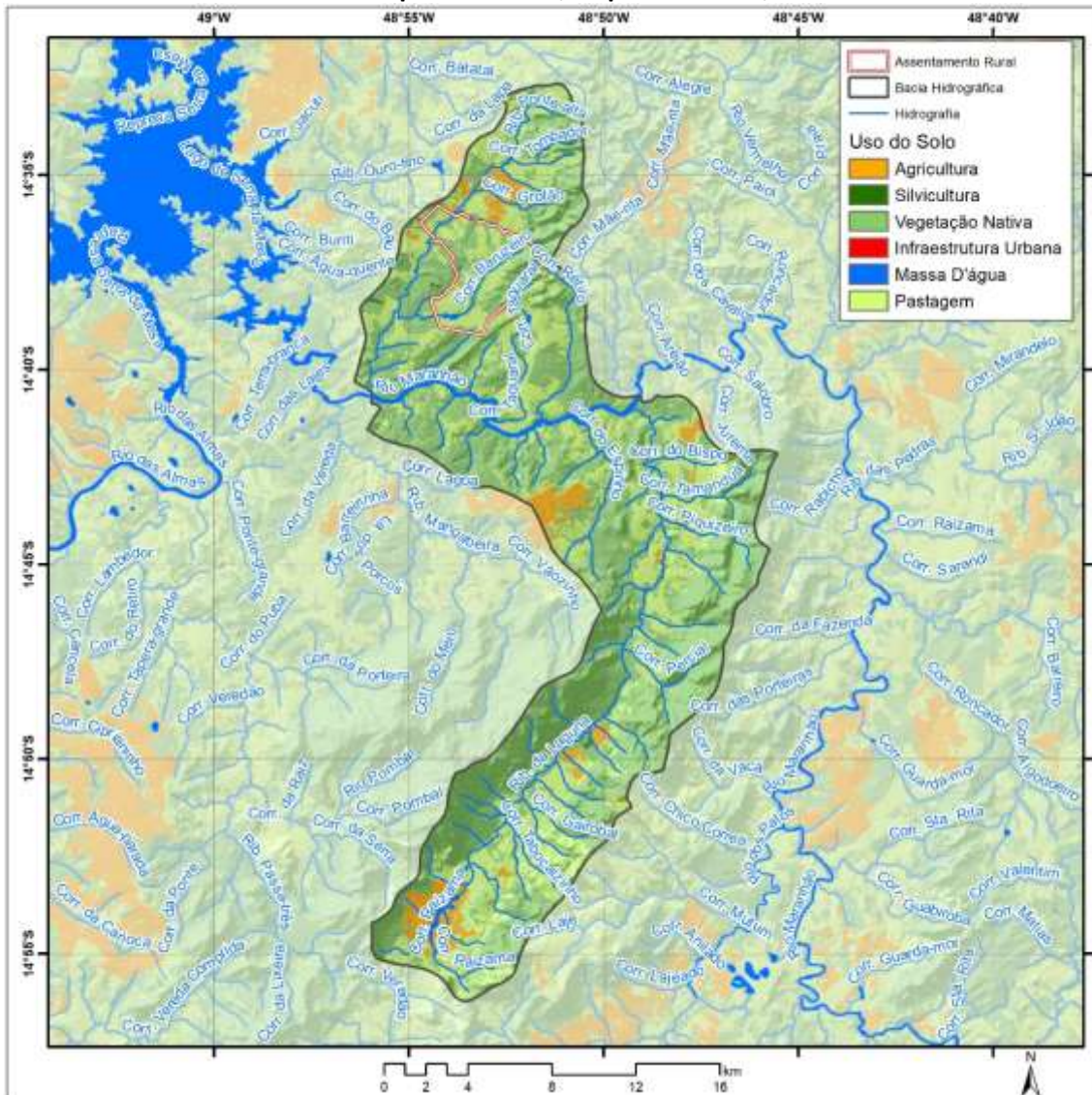
Mapa 3.3 – Cobertura e uso do solo na porção da bacia hidrográfica do rio Maranhão e no assentamento da Comunidade Salto para o Futuro, Niquelândia-GO, 2020.
