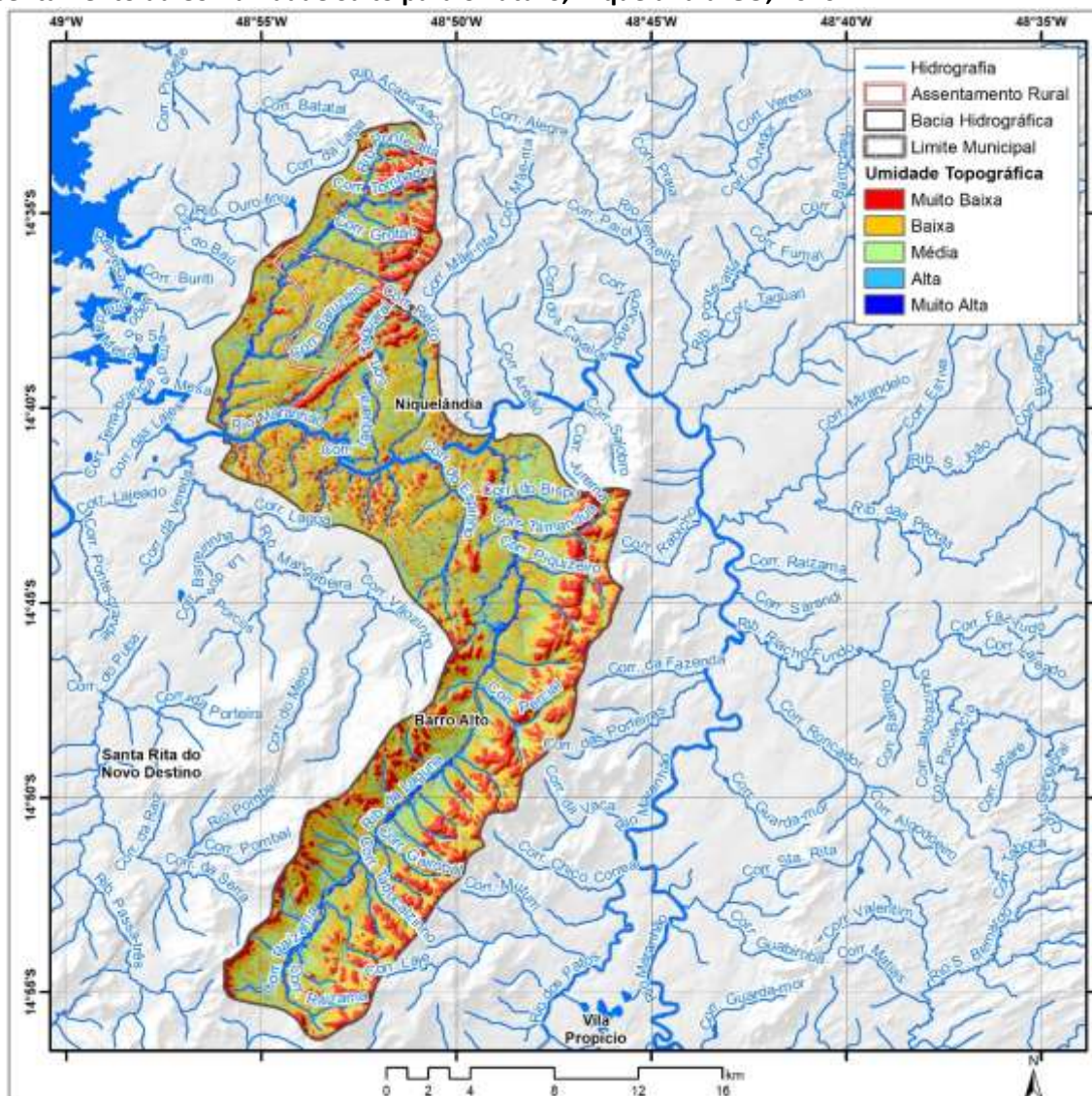
Mapa 3.10 – Índice de umidade topográfica na porção da bacia hidrográfica do rio Maranhão e do assentamento da Comunidade Salto para o Futuro, Niquelândia-GO, 2020.
