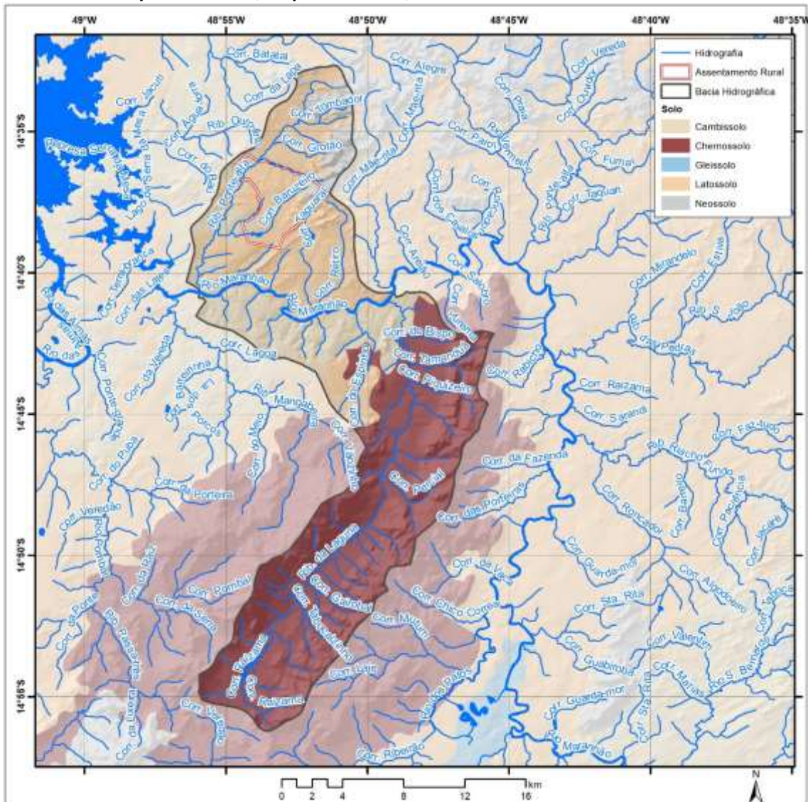
Mapa 3.7 – Tipo de solo da porção da bacia hidrográfica do rio Maranhão e do assentamento da Comunidade Salto para o Futuro, Niquelândia-GO, 2020.
