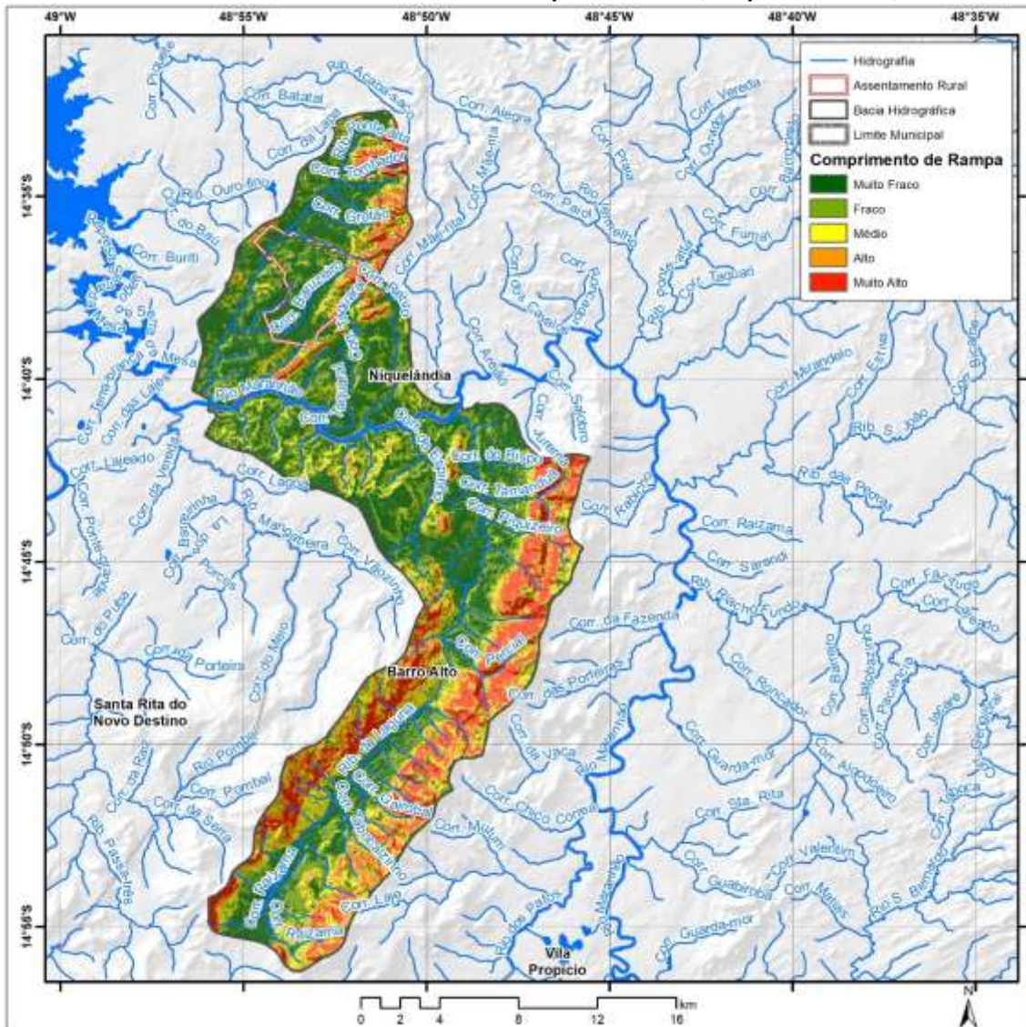
Mapa 3.8 – Comprimento de rampas de declividade do relevo na porção da bacia hidrográfica do rio Maranhão e do assentamento da Comunidade Salto para o Futuro, Niquelândia-GO, 2020.
