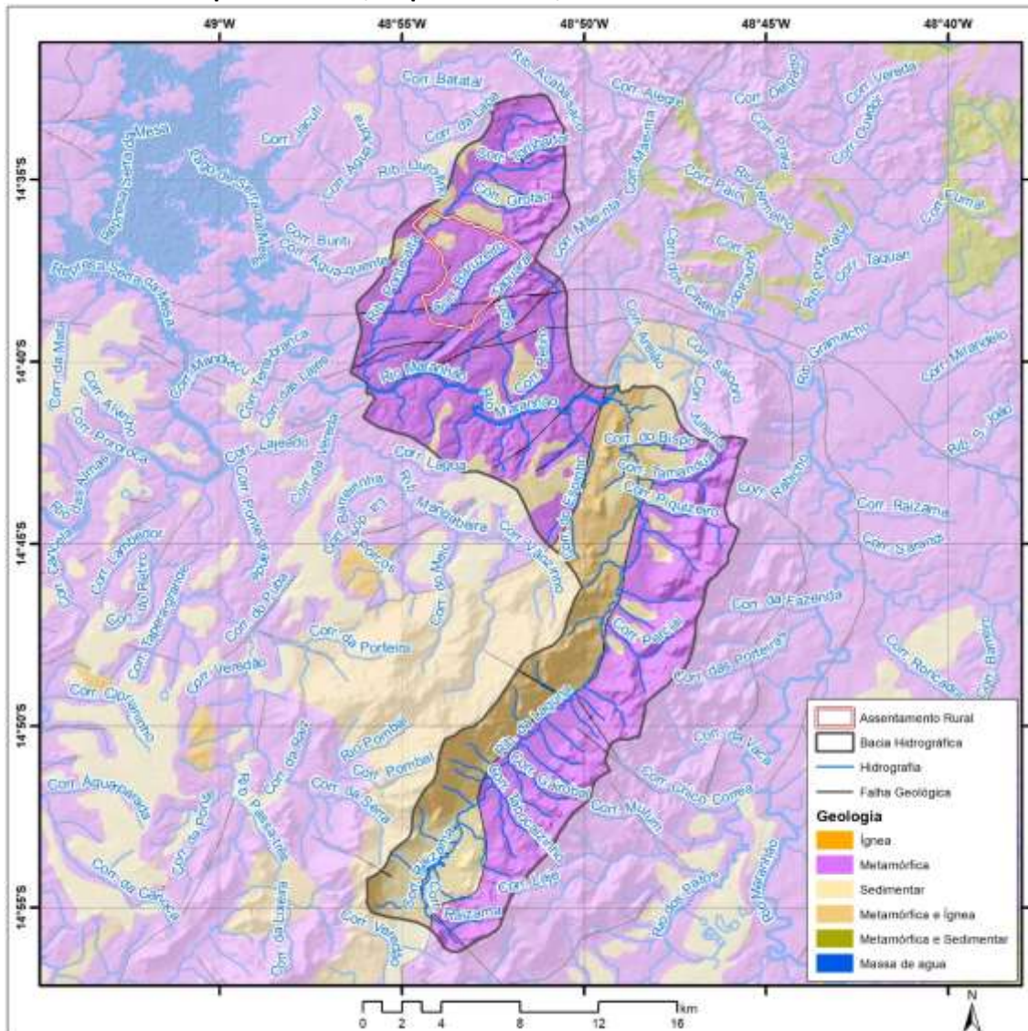
Mapa 3.4 – Litologia da porção da bacia hidrográfica do rio Maranhão e do assentamento da Comunidade Salto para o Futuro, Niquelândia-GO, 2020.
