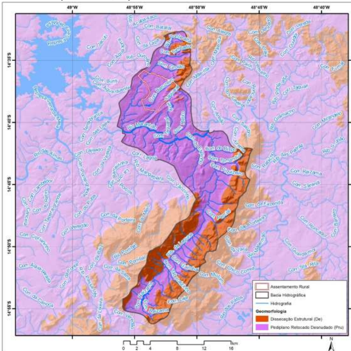
Mapa 3.5 – Geomorfologia da porção da bacia hidrográfica do rio Maranhão e do assentamento da Comunidade Salto para o Futuro, Niquelândia-GO, 2020.
