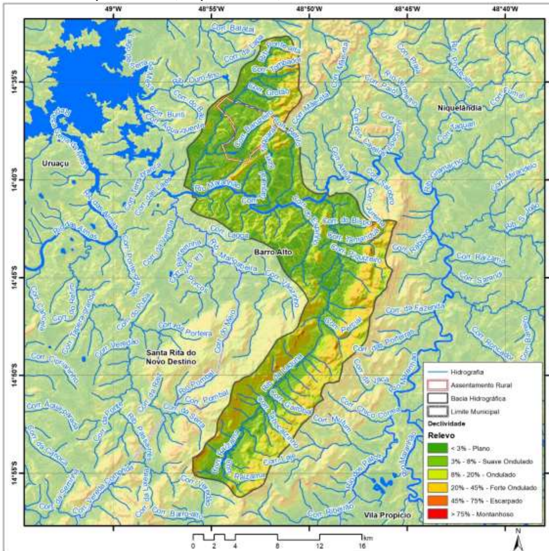
Mapa 3.6 – Declividade da porção da bacia hidrográfica do rio Maranhão e do assentamento da Comunidade Salto para o Futuro, Niquelândia-GO, 2020.
