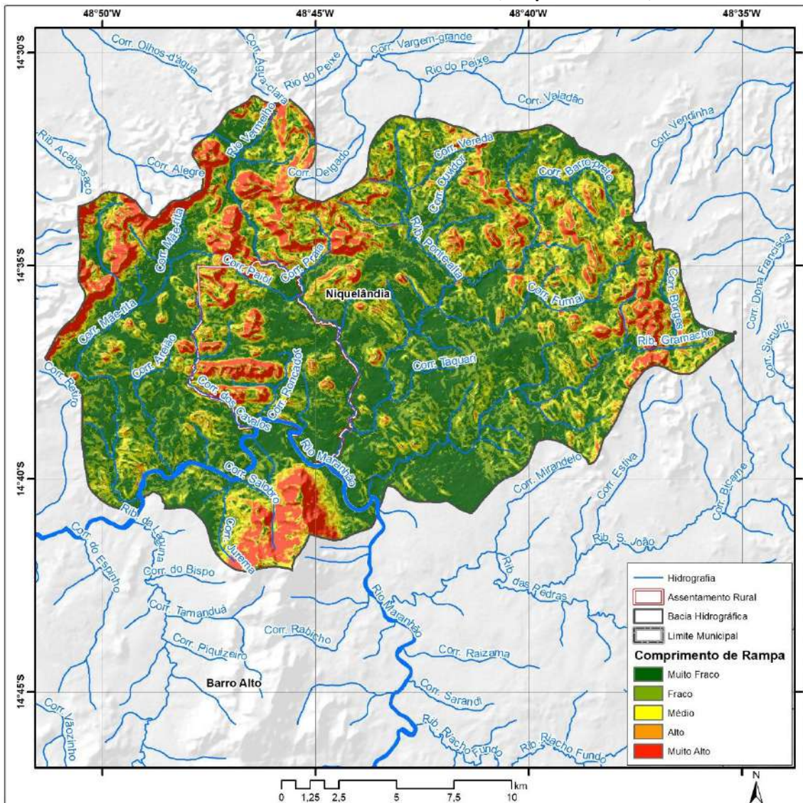
Mapa 3.8 – Comprimento de rampas de declividade do relevo na porção da bacia hidrográfica do rio Maranhão e do assentamento da Comunidade Rio Vermelho, Niquelândia-GO, 2020.
