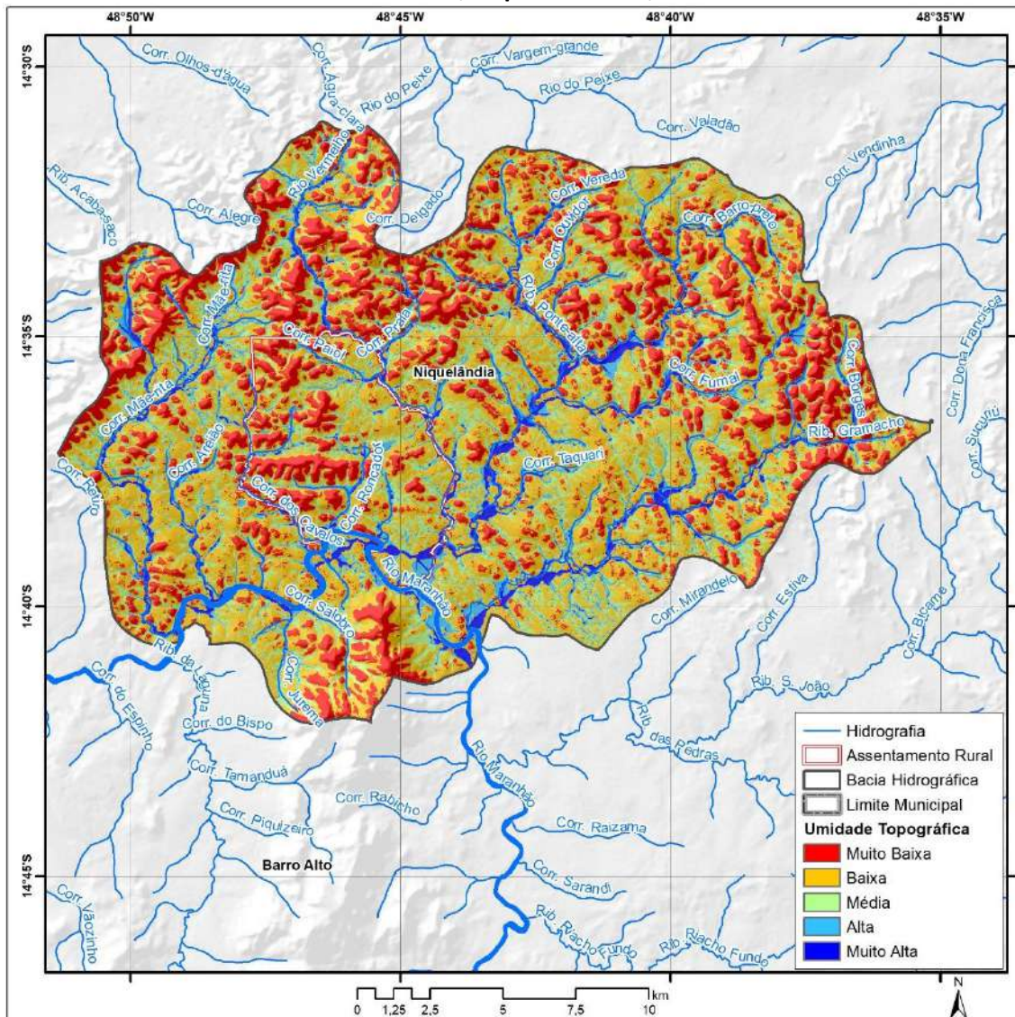
Mapa 3.10 – Índice de umidade topográfica na porção da bacia hidrográfica do rio Maranhão e do assentamento da Comunidade Rio Vermelho, Niquelândia-GO, 2020.
