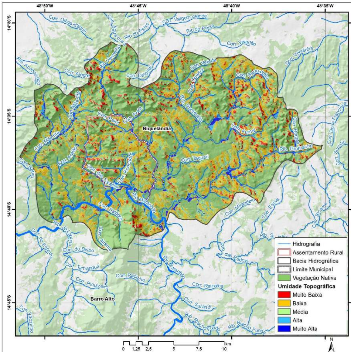
Mapa 3.11 – Índice de umidade topográfica e cobertura de vegetação nativa remanescente na porção da bacia hidrográfica do rio Maranhão e do assentamento da Comunidade Rio Vermelho, Niquelândia-GO, 2020.
