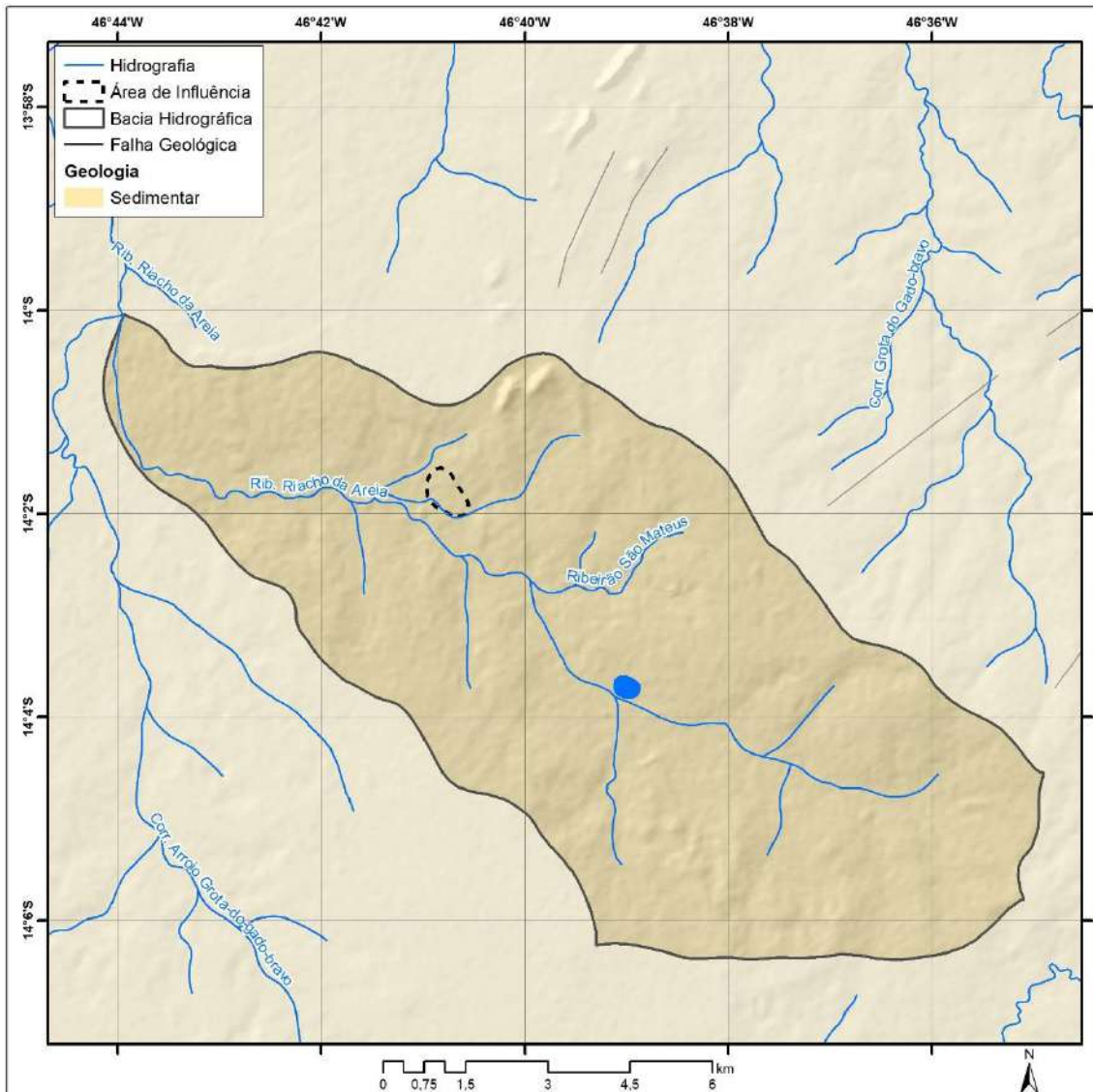
Mapa 3.4 – Litologia da bacia hidrográfica do ribeirão Riacho da Areia e da área de influência da Comunidade de Povoado Levantado, Iaciara-GO, 2020.
