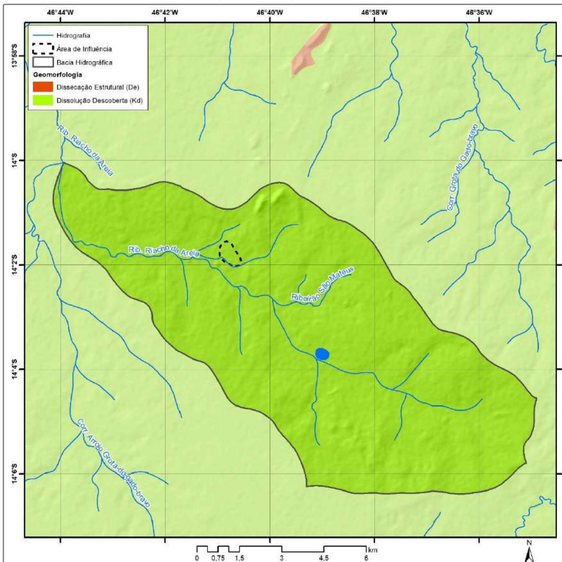
Mapa 3.5 – Geomorfologia da bacia hidrográfica do ribeirão Riacho da Areia e da área de influência da Comunidade de Povoado Levantado, Iaciara-GO, 2020.
