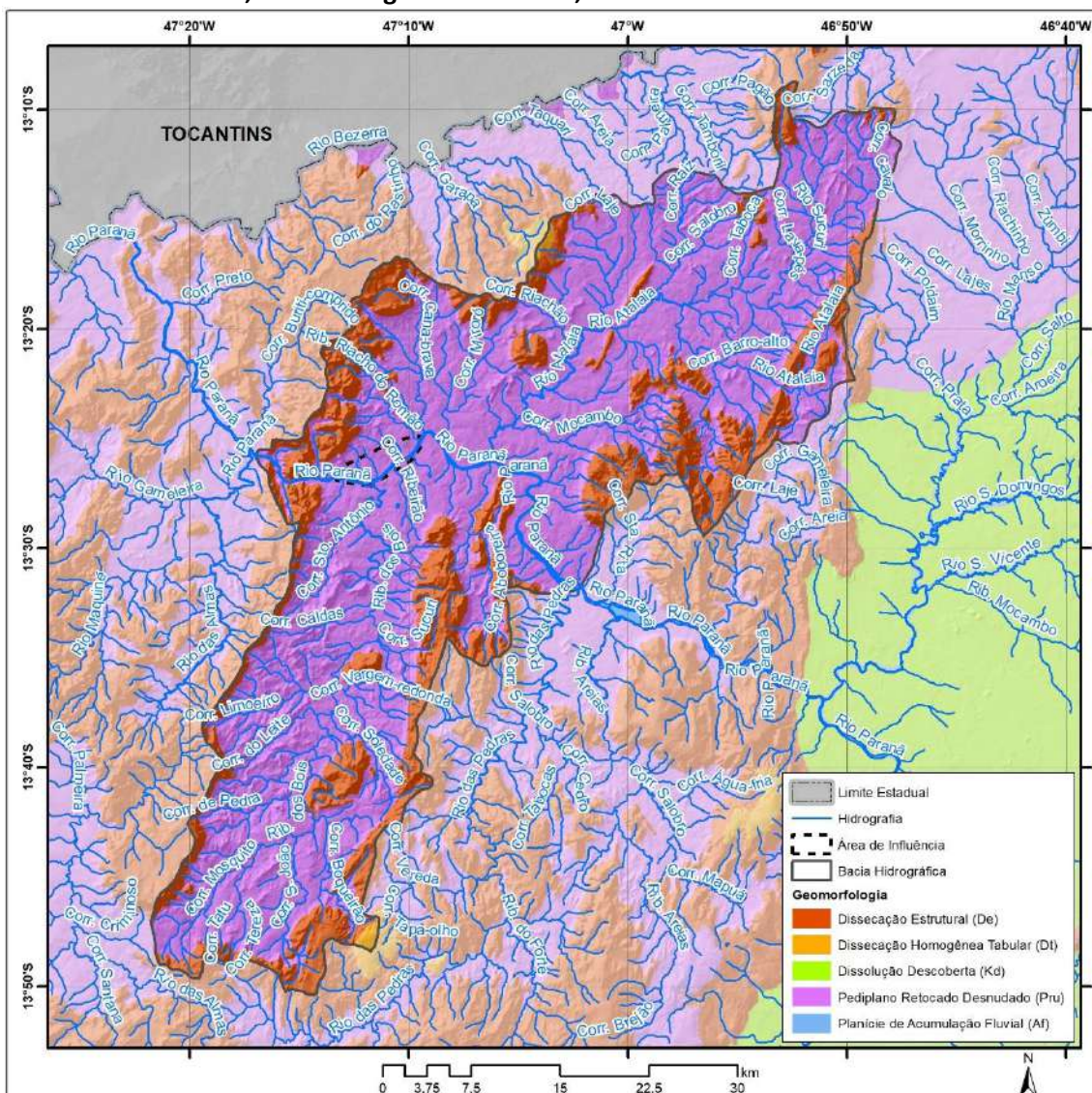
Mapa 3.5 – Geomorfologia da porção da bacia hidrográfica do rio Paranã e da área de influência da Comunidade de Pelotas, Monte Alegre de Goiás-GO, 2020.
