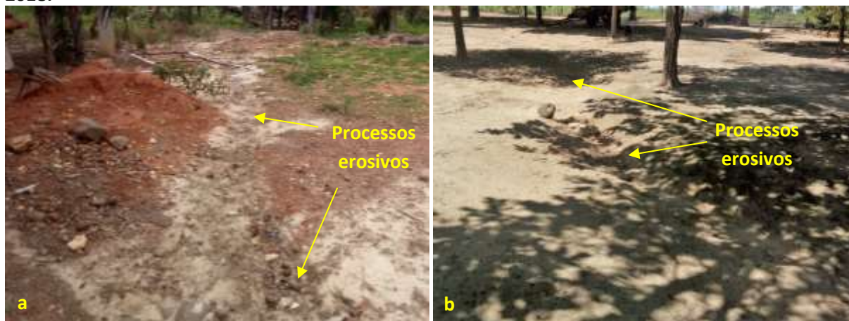
Foto 6.20 – Processos erosivos em lotes da Comunidade Novo Horizonte II, São Luiz do Norte-GO, 2018.
