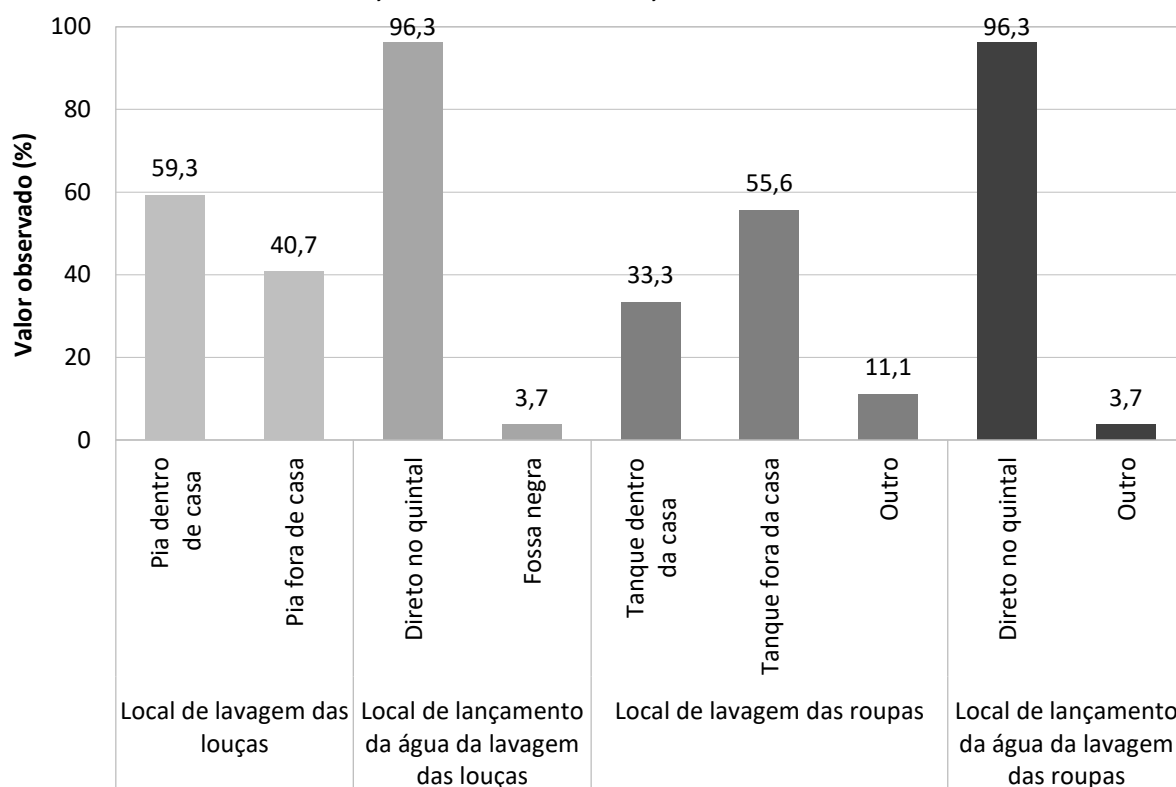
Gráfico 6.4 – Localização dos aparelhos hidrossanitários e locais de geração e de lançamento da água cinza, proveniente da pia para lavagem das louças e do tanque para lavagem das roupas, na Comunidade Novo Horizonte II, São Luiz do Norte-GO, 2018.
