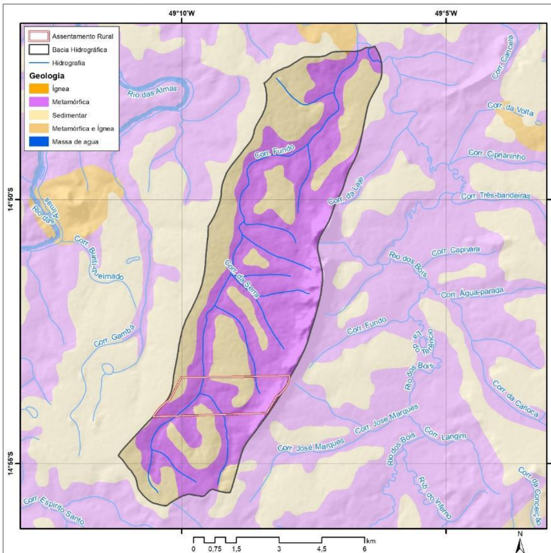
Mapa 3.4 – Litologia da bacia hidrográfica do córrego Fundo e da área do assentamento da Comunidade Monte Moria, São Luiz do Norte-GO, 2020.
