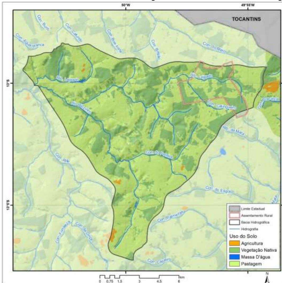
Mapa 3.3 – Cobertura e uso do solo nas bacias hidrográficas do rio Riozinho e do ribeirão Lageado.
