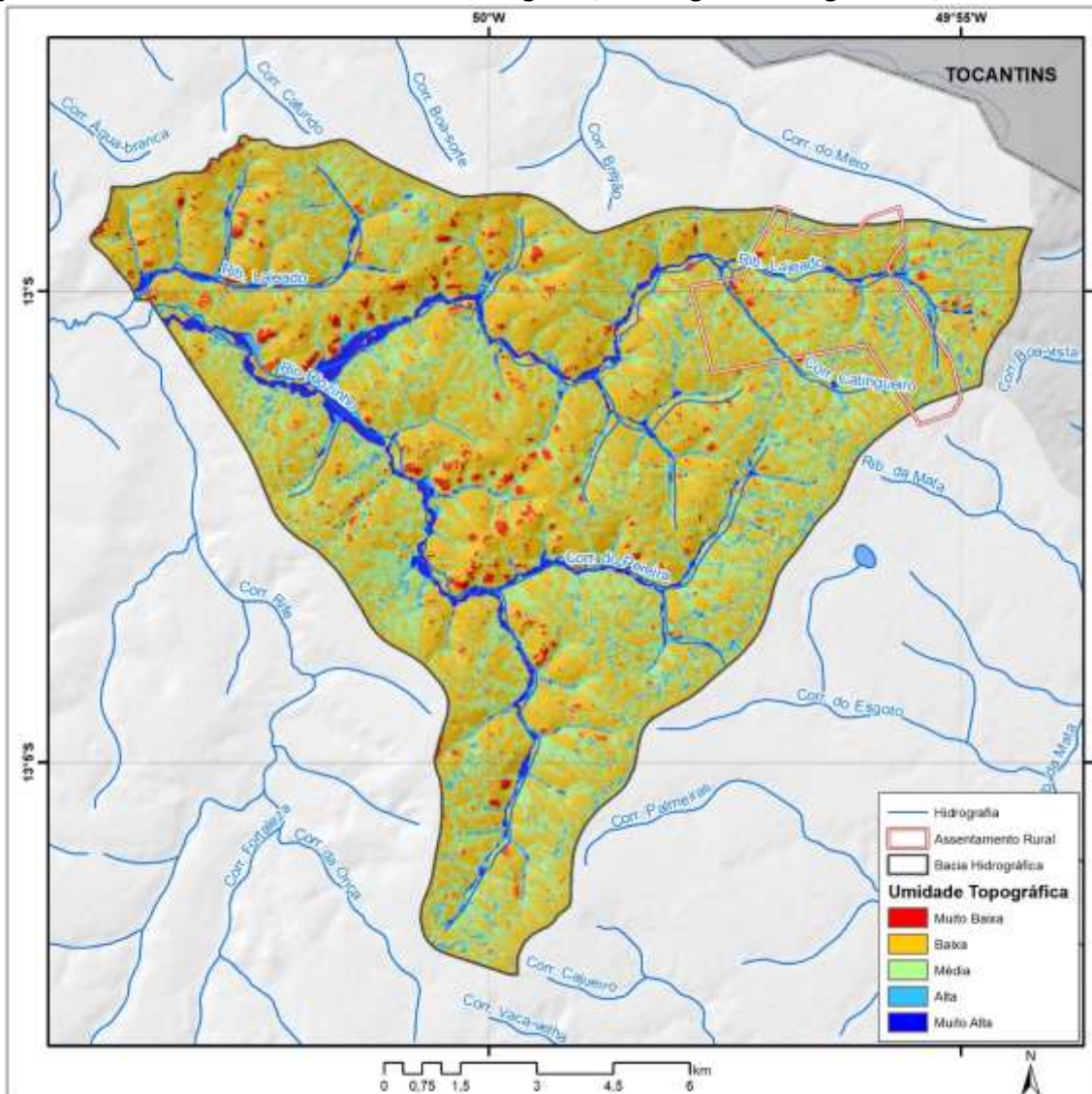
Mapa 3.10 – Índice de umidade topográfica nas bacias hidrográficas do rio Riozinho e do ribeirão Lageado e do assentamento da Comunidade Lageado, São Miguel do Araguaia-GO, 2020.
