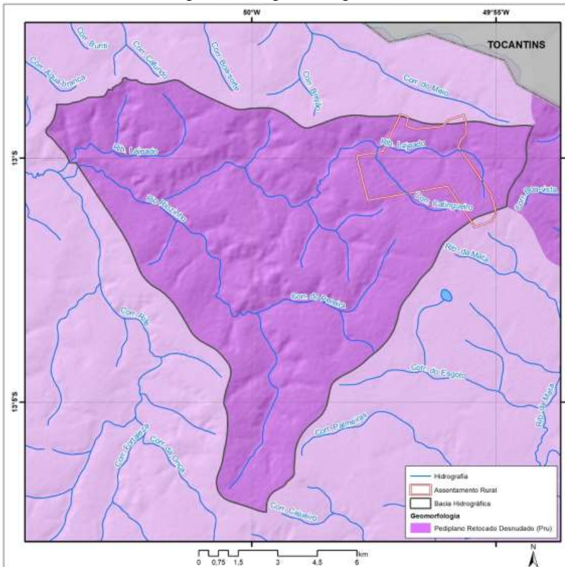
Mapa 3.5 – Geomorfologia das bacias hidrográficas do rio Riozinho e do ribeirão Lageado e do assentamento da Comunidade Lageado, São Miguel do Araguaia-GO, 2020.
