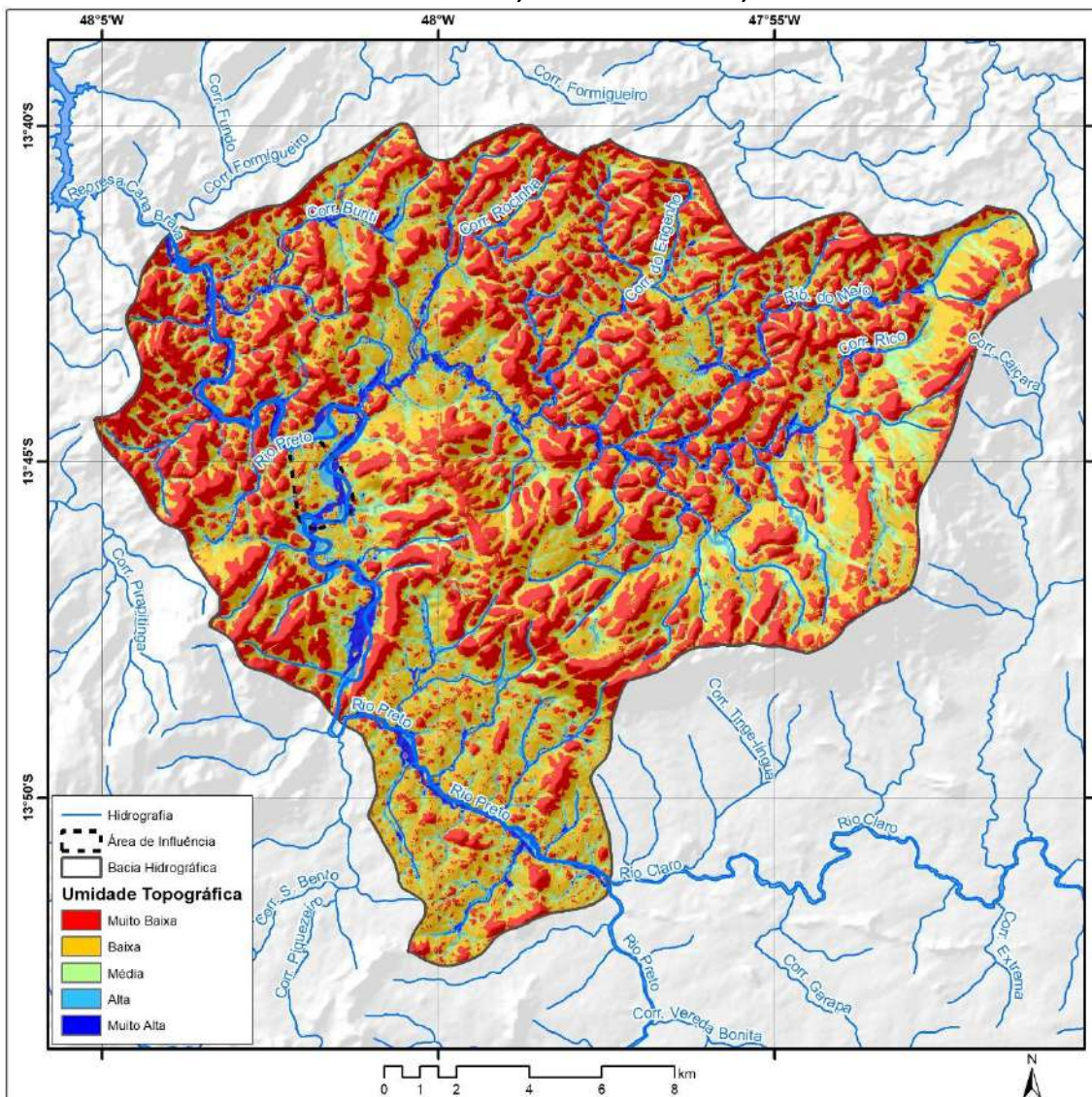
Mapa 3.10 – Índice de umidade topográfica na porção da bacia hidrográfica do rio Preto e da área do território da Comunidade de José de Coletto, Colinas do Sul-GO, 2020.
