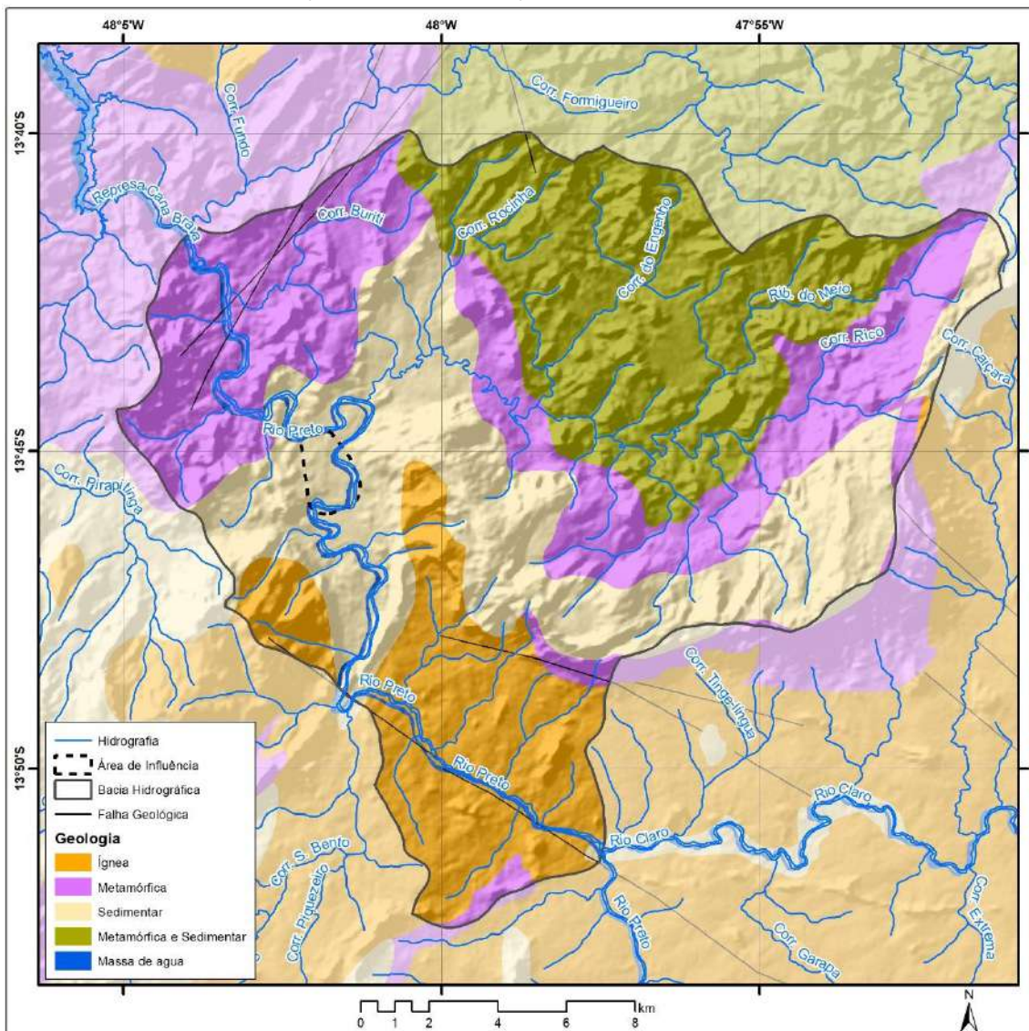
Mapa 3.4 – Litologia da porção da bacia hidrográfica do rio Preto e da área do território da Comunidade de José de Coletto, Colinas do Sul-GO, 2020.
