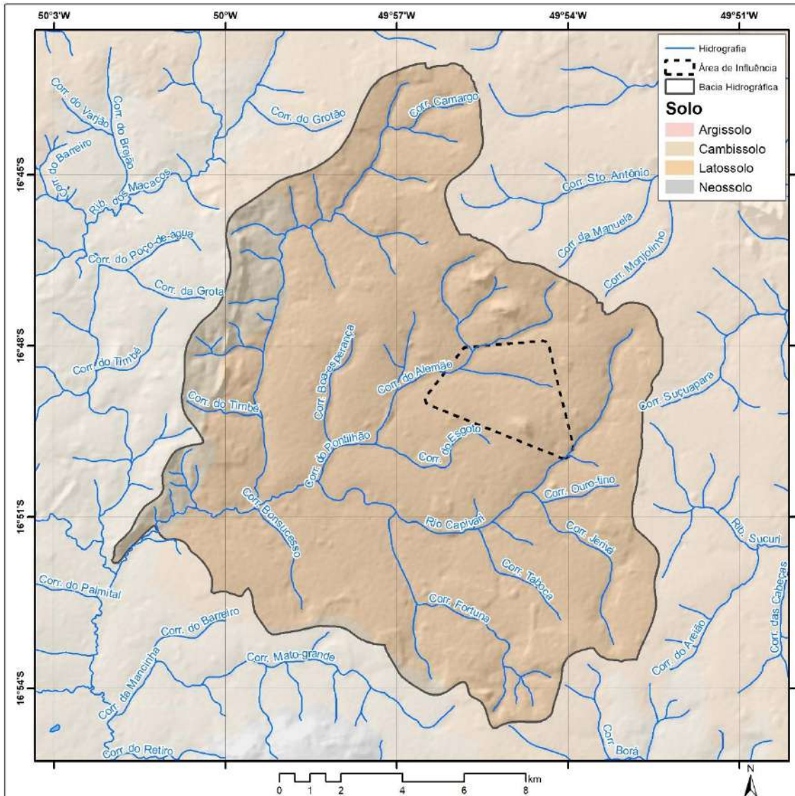
Mapa 3.7 – Tipo de solo da bacia hidrográfica do córrego Pontilhão e da área de influência da Comunidade Goianinha, Palmeiras de Goiás-GO, 2020.
