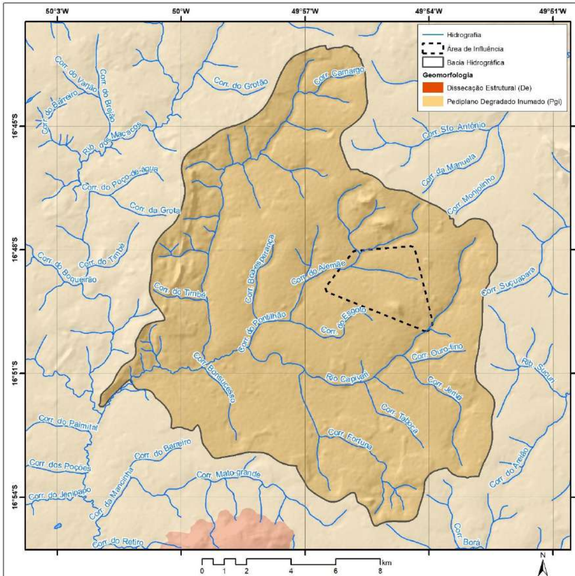
Mapa 3.5 – Geomorfologia da bacia hidrográfica do córrego Pontilhão e da área de influência da Comunidade Goianinha, Palmeiras de Goiás-GO, 2020.
