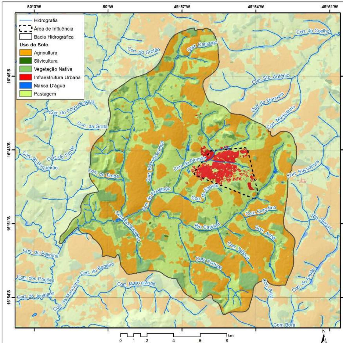
Mapa 3.3 – Cobertura e uso do solo na bacia hidrográfica do córrego Pontilhão e da área de influência da Comunidade Goianinha, Palmeiras de Goiás-GO, 2020.
