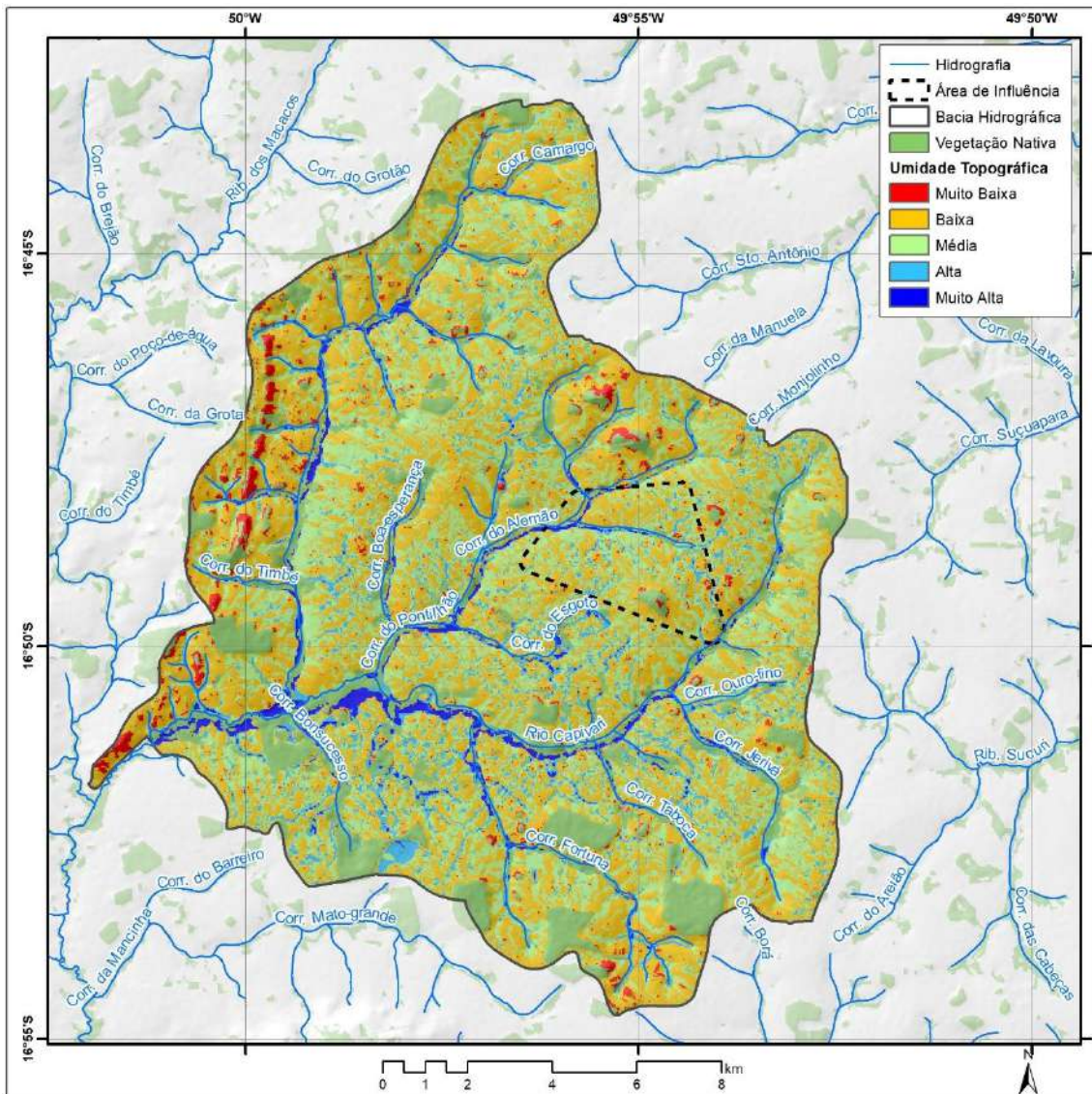
Mapa 3.11 – Índice de umidade topográfica e cobertura de vegetação nativa remanescente na bacia hidrográfica do córrego Pontilhão e da área de influência da Comunidade Goianinha, Palmeiras de Goiás-GO, 2020.
