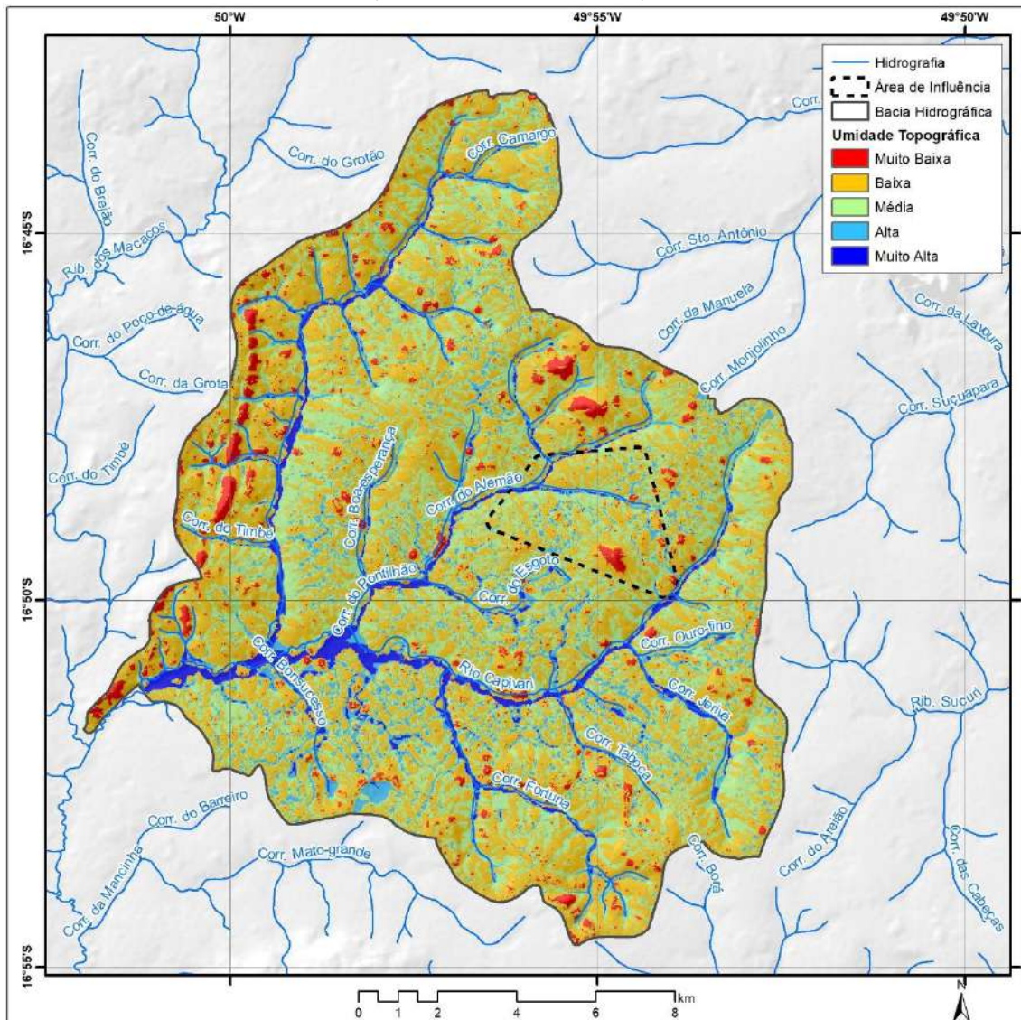
Mapa 3.10 – Índice de umidade topográfica na bacia hidrográfica do córrego Pontilhão e da área de influência da Comunidade Goianinha, Palmeiras de Goiás-GO, 2020.
