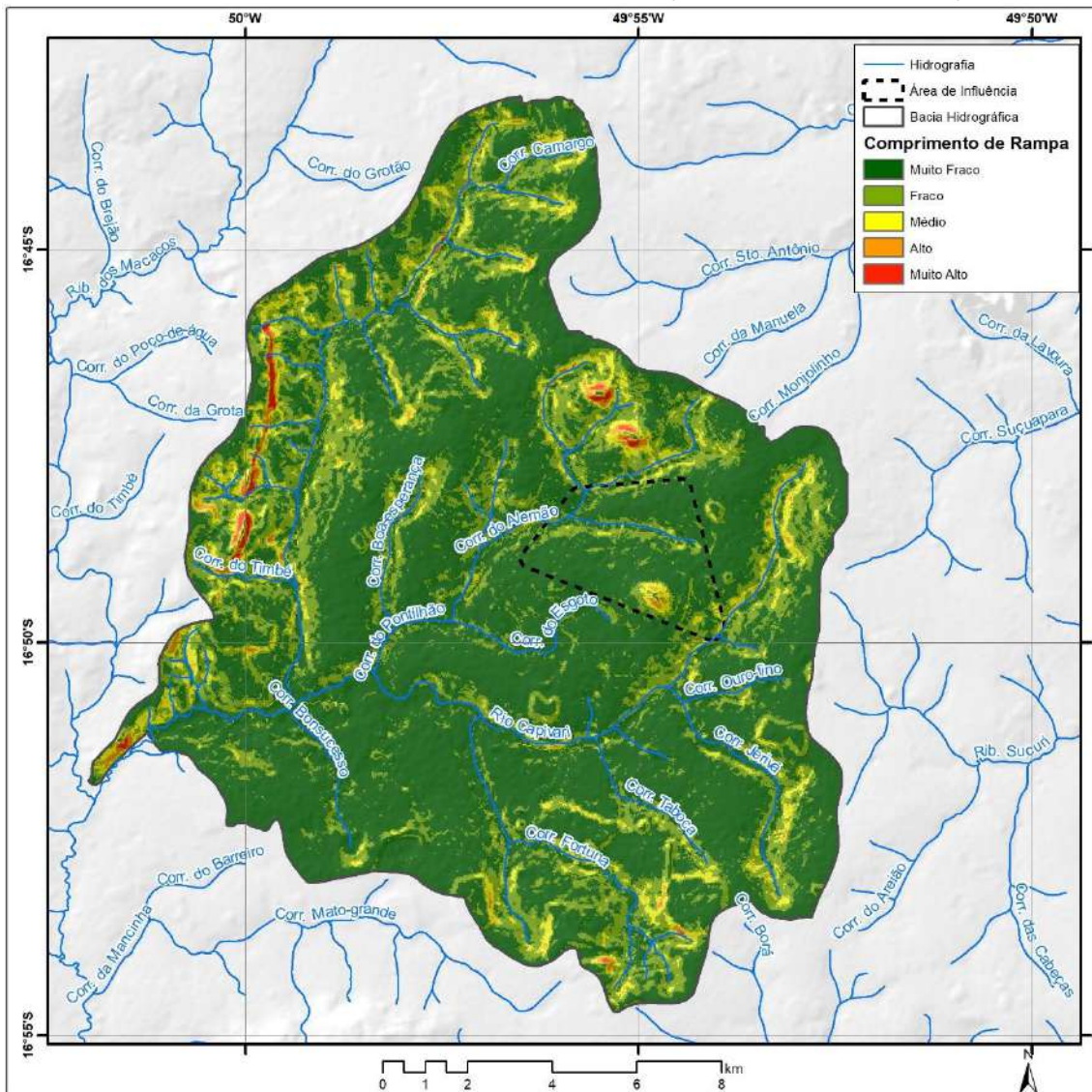
Mapa 3.8 – Comprimento de rampas de declividade do relevo na bacia hidrográfica do córrego Pontilhão e da área de influência da Comunidade Goianinha, Palmeiras de Goiás-GO, 2020.
