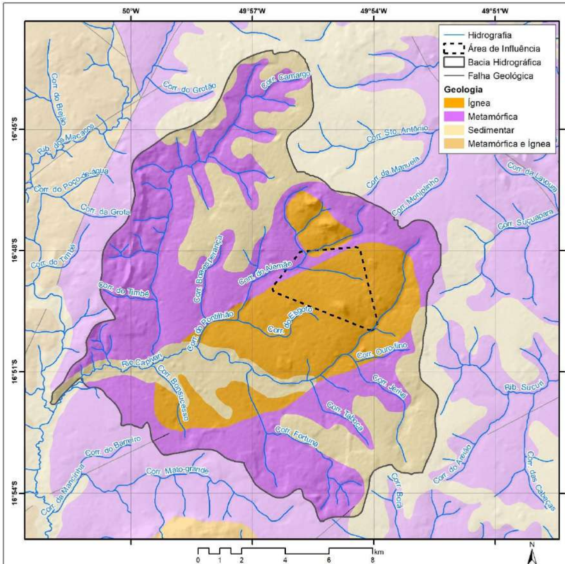
Mapa 3.4 – Litologia da bacia hidrográfica do córrego Pontilhão e da área de influência da Comunidade Goianinha, Palmeiras de Goiás-GO, 2020.
