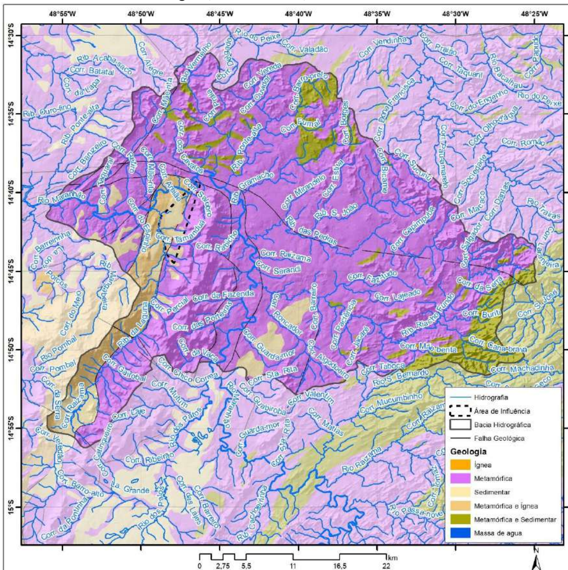
Mapa 3.4 – Litologia da bacia hidrográfica do rio Maranhão e da área de influência da Comunidade da Fazenda Santo Antônio da Laguna, Barro Alto-GO, 2020.
