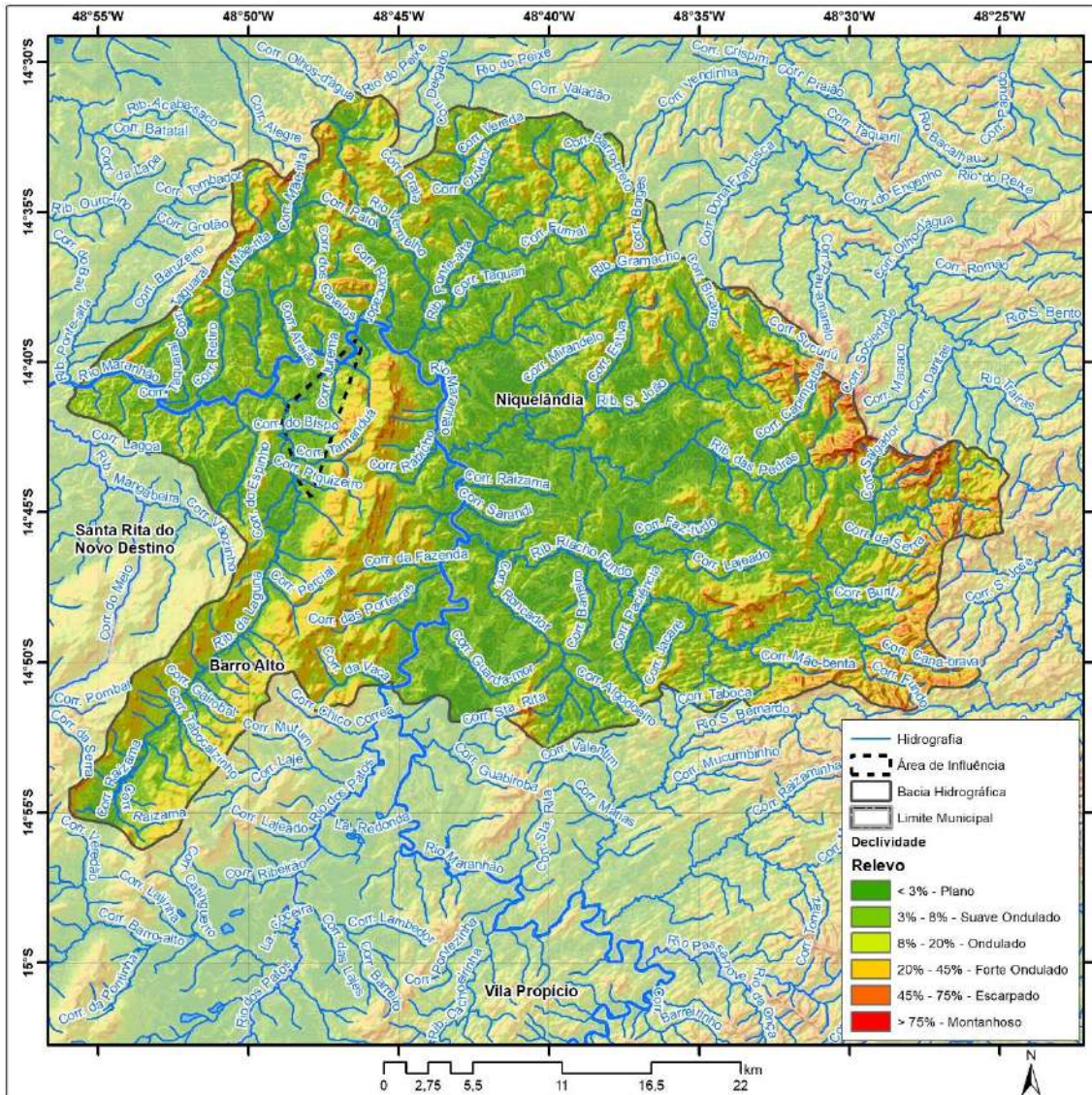
Mapa 3.6 – Declividade da bacia hidrográfica do rio Maranhão e da área de influência da Comunidade da Fazenda Santo Antônio da Laguna, Barro Alto-GO, 2020.
