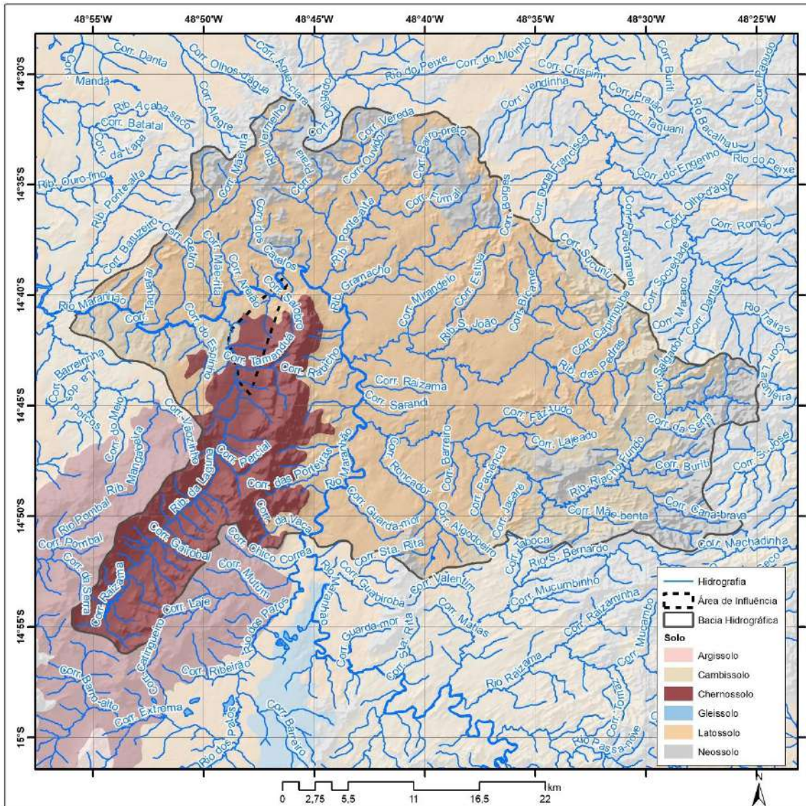
Mapa 3.7 – Tipos de solos da bacia hidrográfica do rio Maranhão e da área de influência da Comunidade da Fazenda Santo Antônio da Laguna, Barro Alto-GO, 2020.
