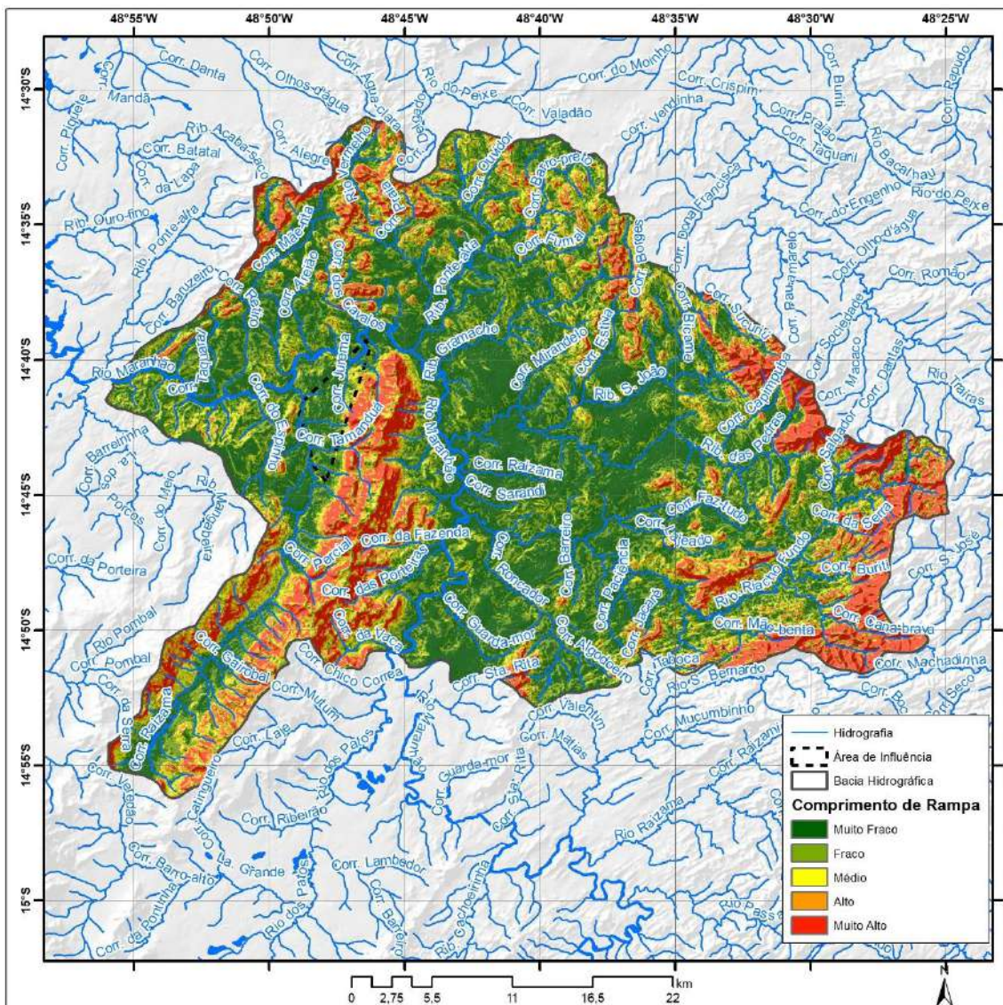
Mapa 3.8 – Comprimentos de rampas de declividades dos relevos na bacia hidrográfica do rio Maranhão e da área de influência Comunidade da Fazenda Santo Antônio da Laguna, Barro Alto-GO, 2020.
