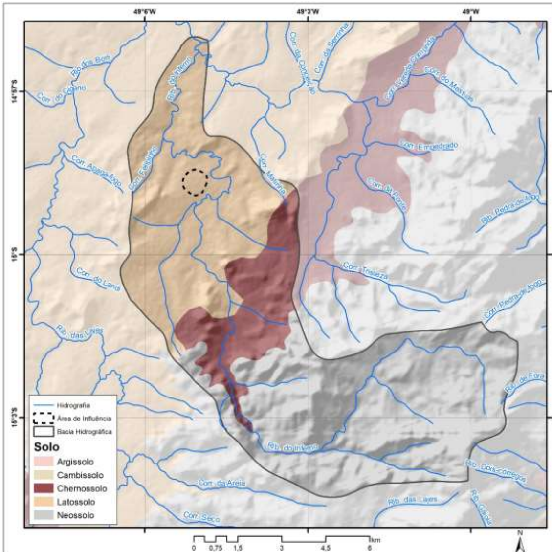
Mapa 3.7 – Tipo de solo da bacia hidrográfica do ribeirão Inferno e da área de influência da Comunidade de Balbino dos Santos, Santa Rita do Novo Destino-GO, 2020.
