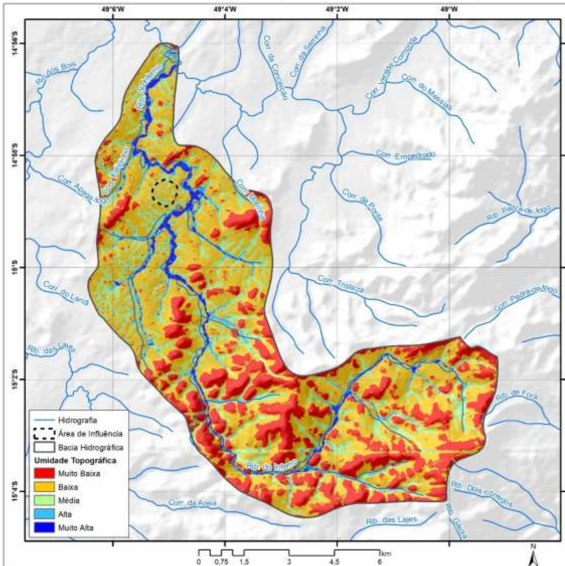
Mapa 3.10 – Índice de umidade topográfica na bacia hidrográfica do ribeirão Inferno e da área de influência da Comunidade de Balbino dos Santos, Santa Rita do Novo Destino-GO, 2020.
