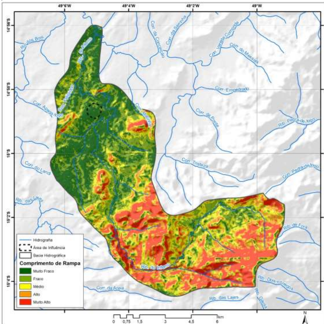
Mapa 3.8 – Comprimento de rampas de declividade do relevo na bacia hidrográfica do ribeirão Inferno e da área de influência da Comunidade de Balbino dos Santos, Santa Rita do Novo Destino-GO, 2020.
