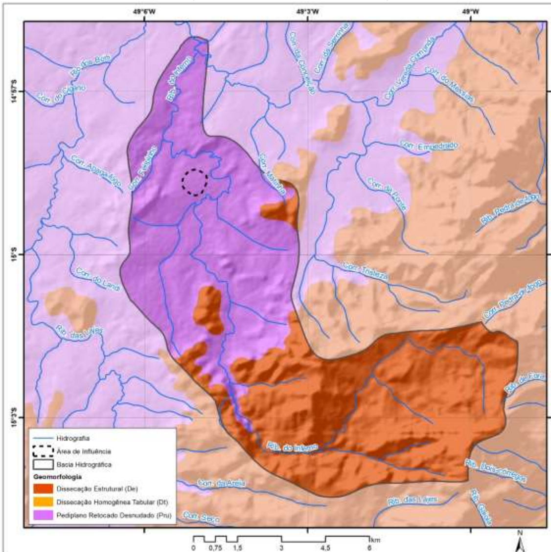
Mapa 3.5 – Geomorfologia da bacia hidrográfica do ribeirão Inferno e da área de influência da Comunidade de Balbino dos Santos, Santa Rita do Novo Destino-GO, 2020.
