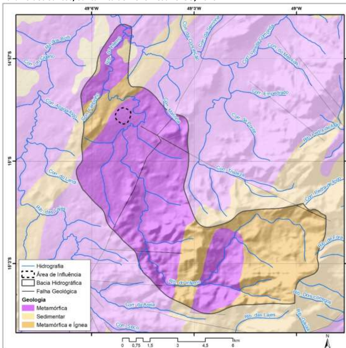
Mapa 3.4 – Litologia da bacia hidrográfica do ribeirão Inferno e da área de influência da Comunidade de Balbino dos Santos, Santa Rita do Novo Destino-GO, 2020.
