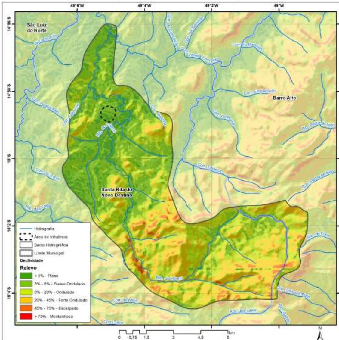
Mapa 3.6 – Declividade da bacia hidrográfica do ribeirão Inferno e da área de influência da Comunidade de Balbino dos Santos, Santa Rita do Novo Destino-GO, 2020.
