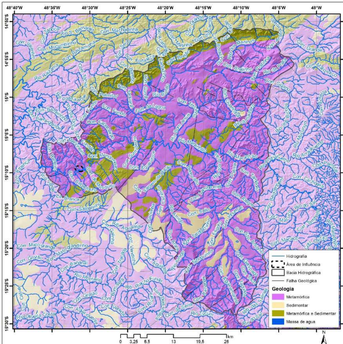
Mapa 3.4 – Litologia da porção da bacia hidrográfica do rio Maranhão e da área do território da Comunidade de Mimoso (Queixo Dantas), Mimoso de Goiás-GO, 2020.
