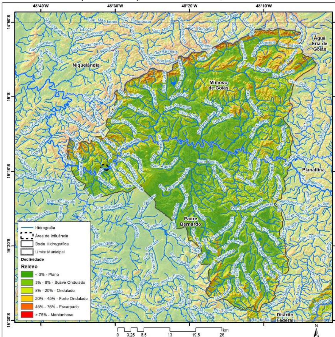
Mapa 3.6 – Declividade da porção da bacia hidrográfica do rio Maranhão e da área do território da Comunidade de Mimoso (Queixo Dantas), Mimoso de Goiás-GO, 2020.
